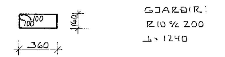
SNID I SÚLU S3 1:20
