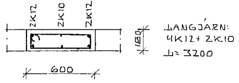
SNID A-A 1:20 SNID B-B 1:20 SNID C-C 1:20 SNID D-D 1:20 SNID E-E 1:20
