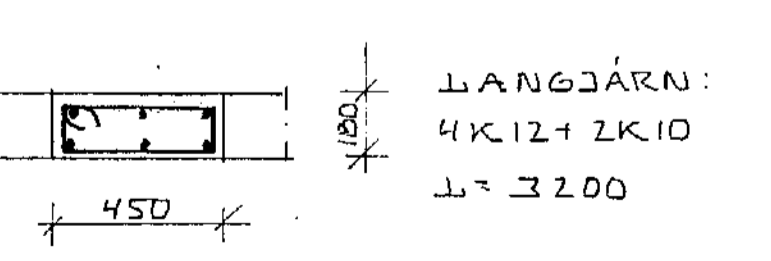
SNID I SÚLU S3 1:20
