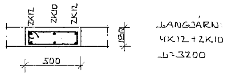
SNID I SÚLU S1 1:20
