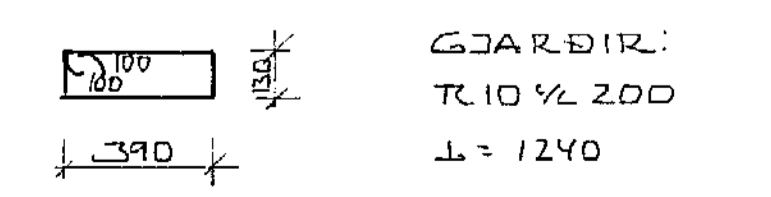
SNID I SÚLU S4 1:20
