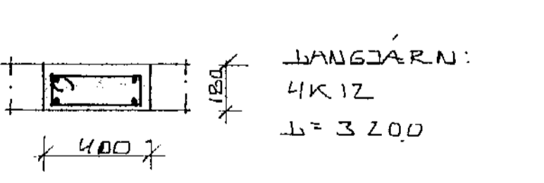
SNID I SÚLU S5 1:20
