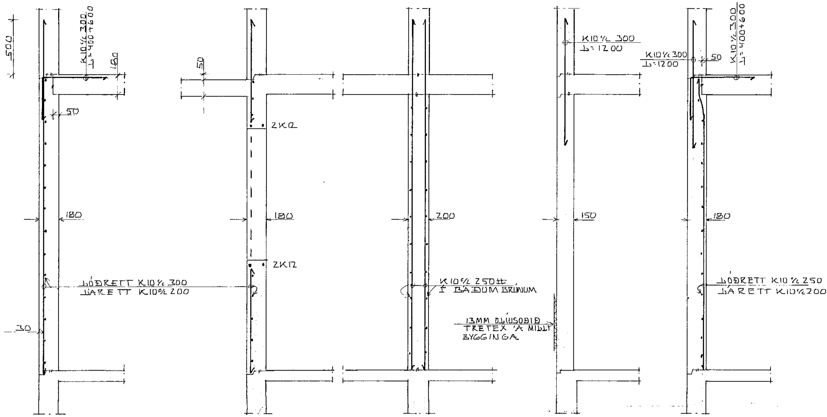
SNID A-A 1:20 SNID B-B 1:20 SNID C-C 1:20 SNID D-D 1:20 SNID E-E 1:20
