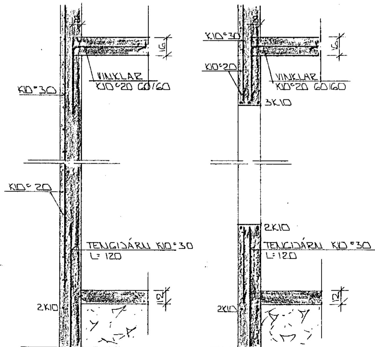
SNID X • 1:20
