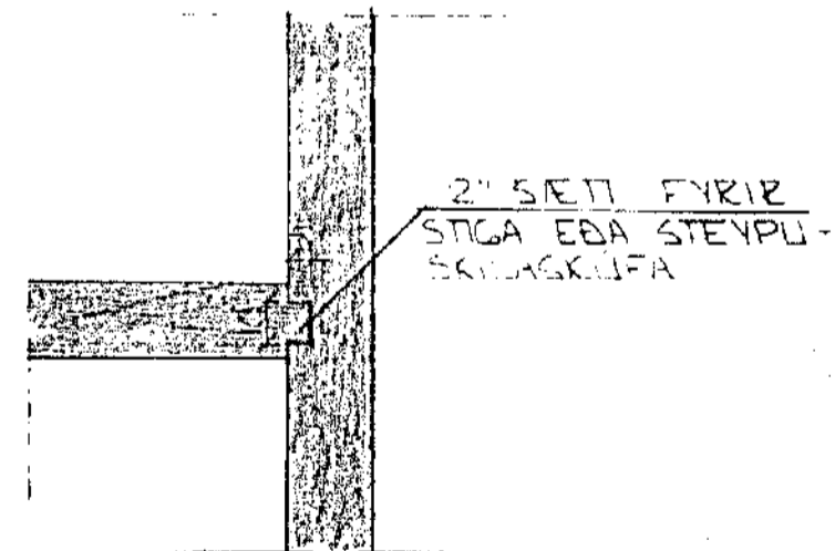
SNID 9 • 1:20
