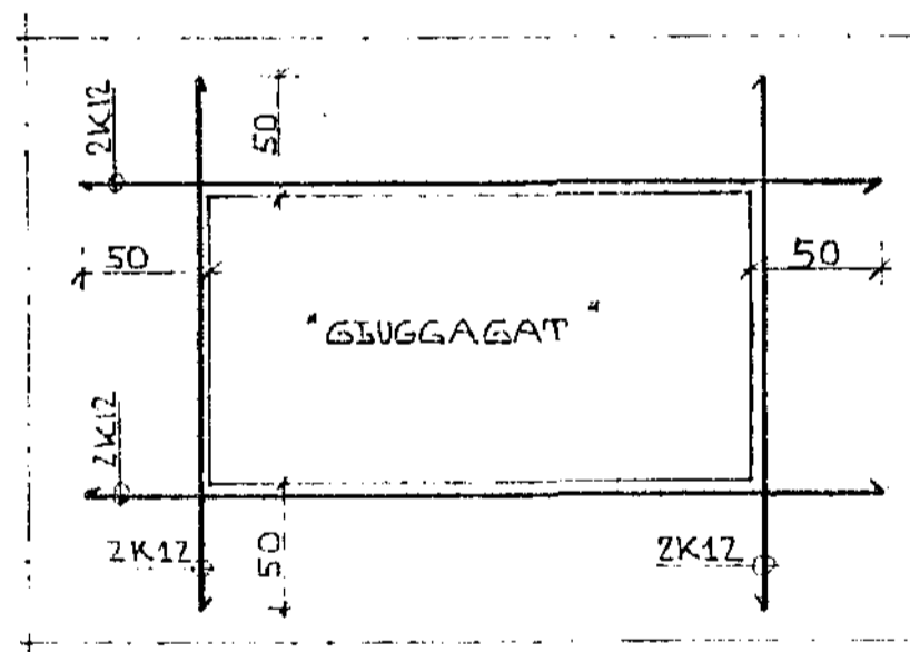
JARN KRINGUM GIUGGA EÐA DYR NEMA ANNAD SÉ SYNT Á TEIKNINGUM
