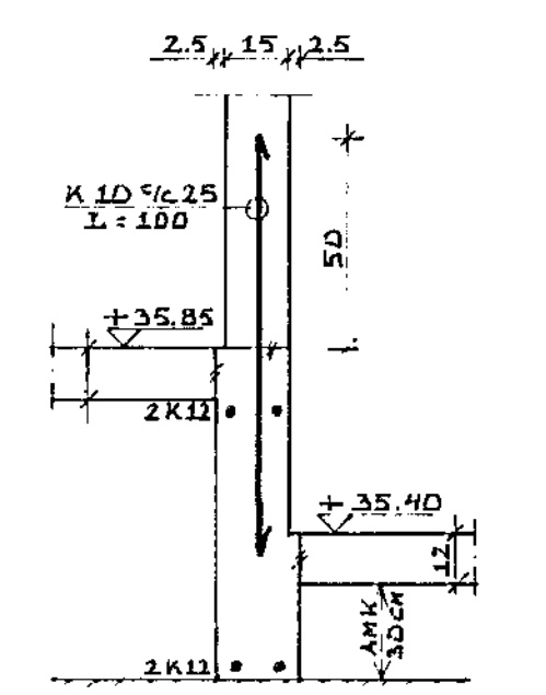
SNID D-D 1:20
