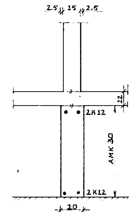
SNID B-B 1:20
