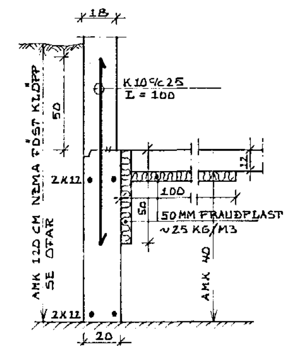
SNID A-A 1:20
