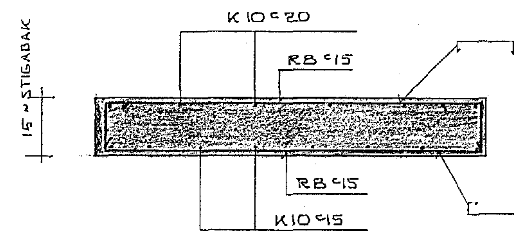
SNID A-A 1:10
