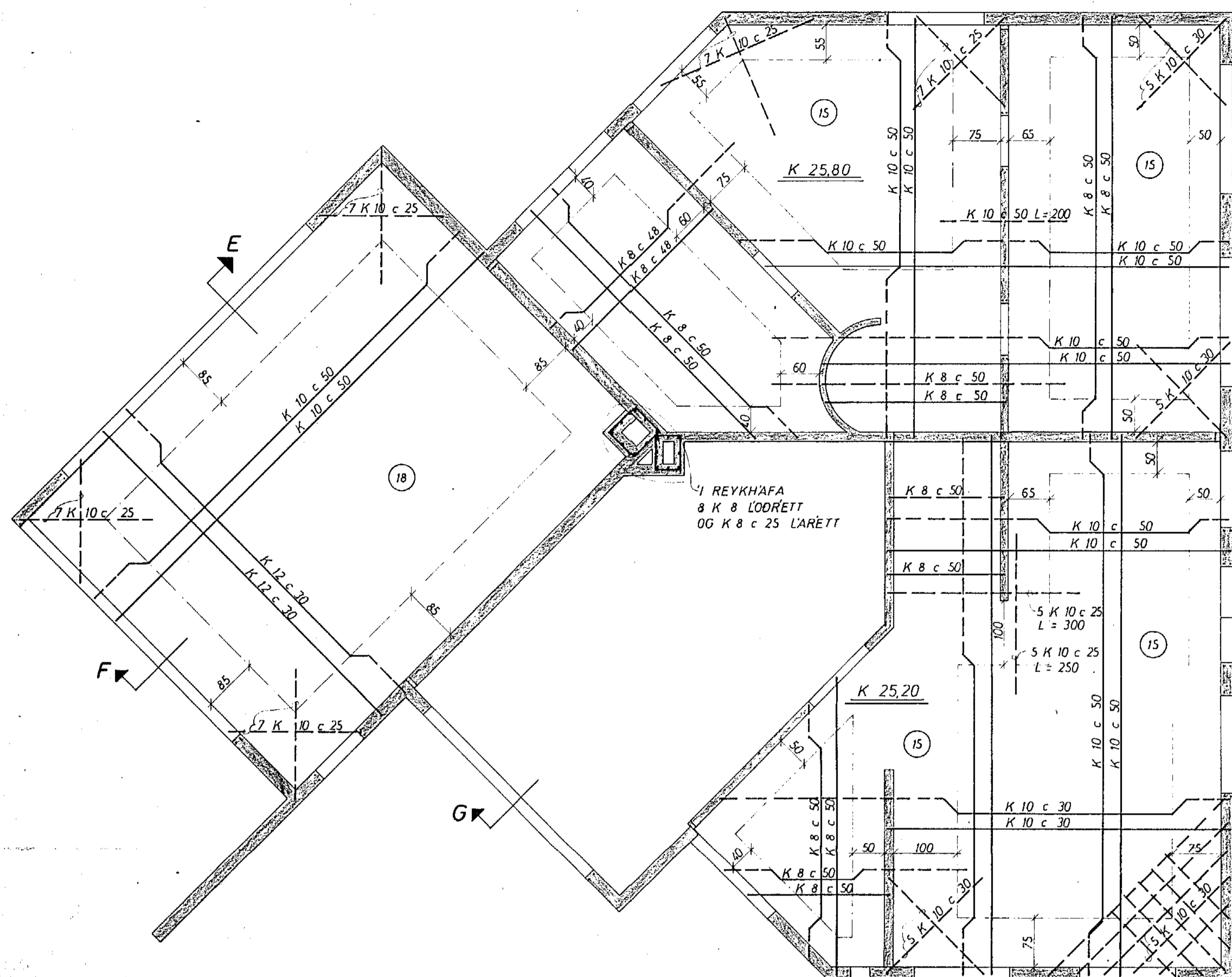
PLATA YFIR 1 HÆÐ 1:50
