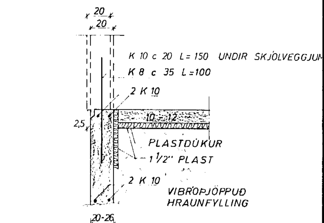
SNID 1 ÚTVEGGI 1:20
