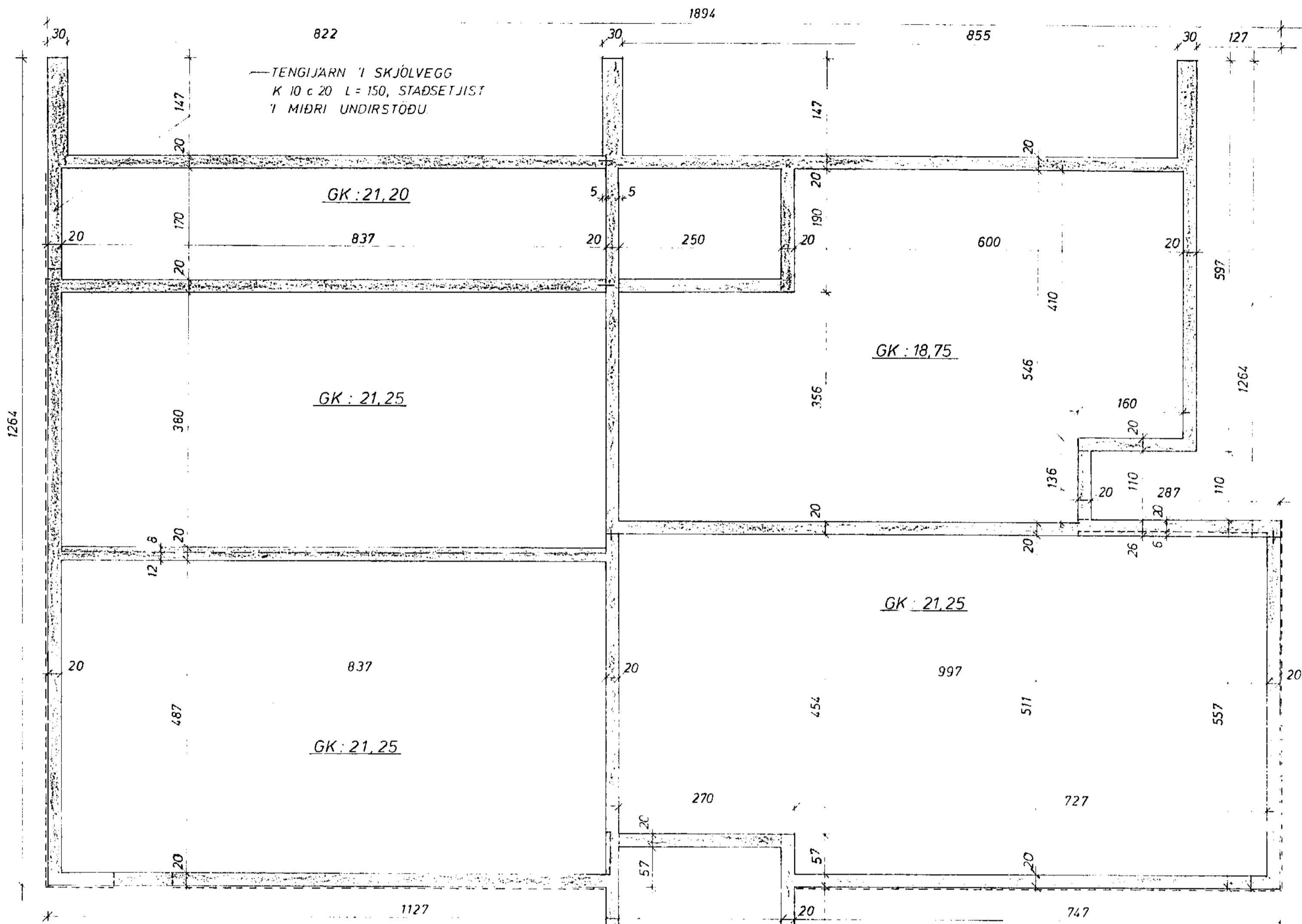
GRUNNMYND 1:50
