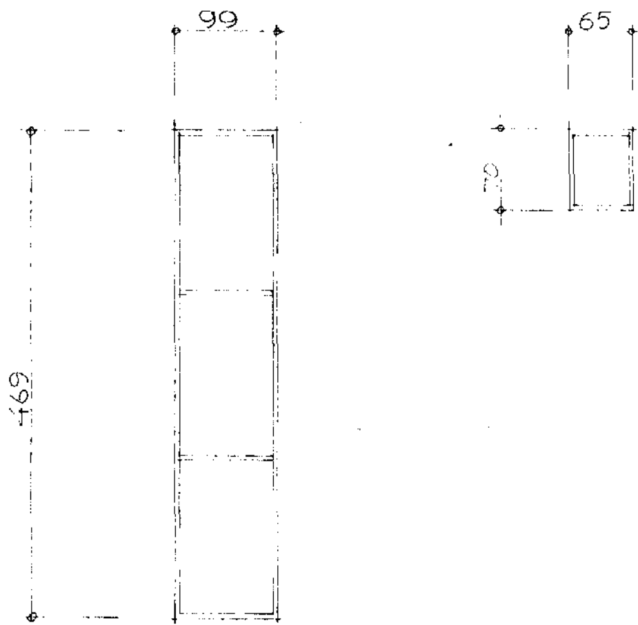
ÚTLIT M 1:50
