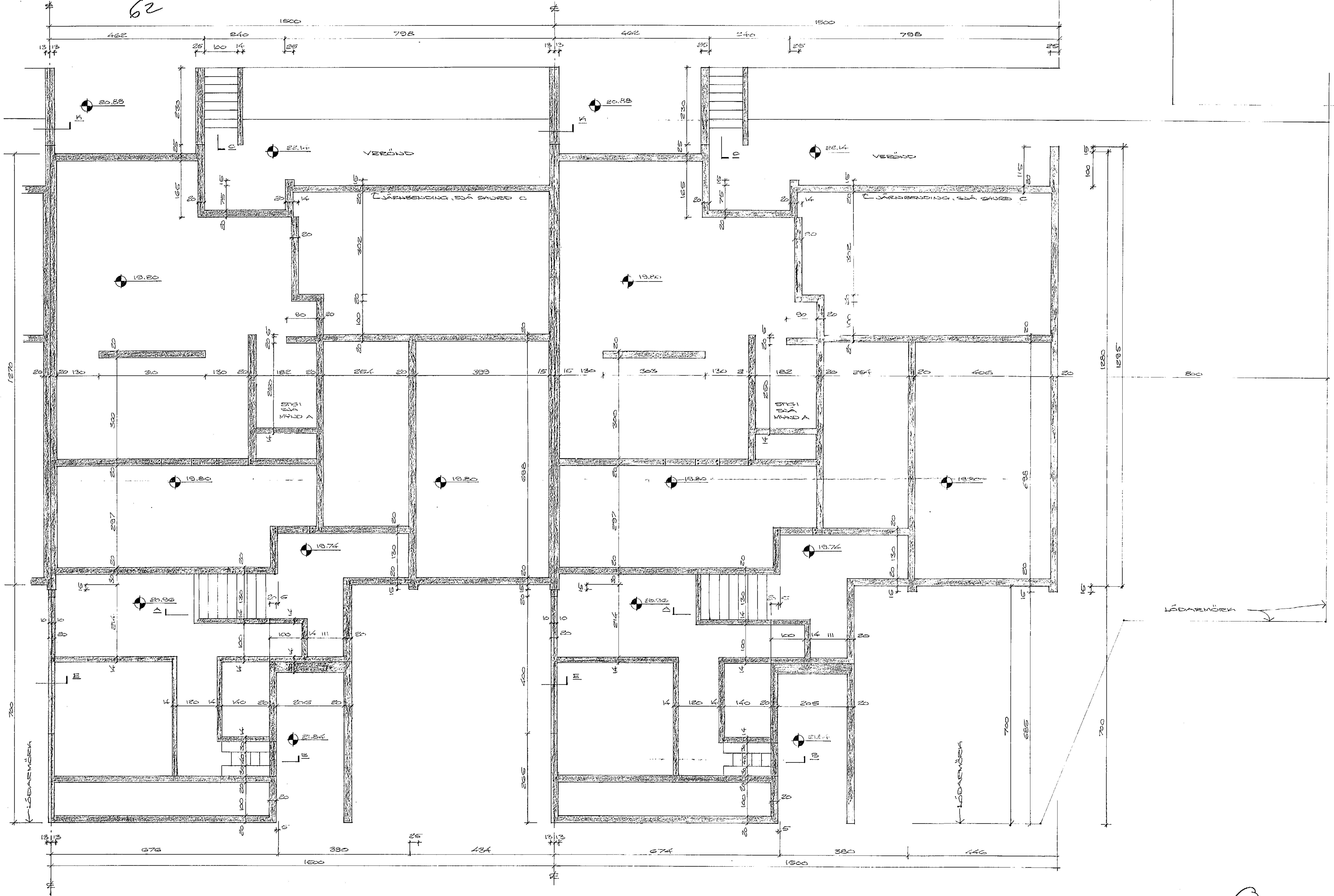
GRUNDMÄTT M. 1:200
