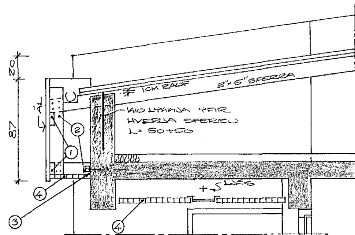
SKURÐUR A, M.182
