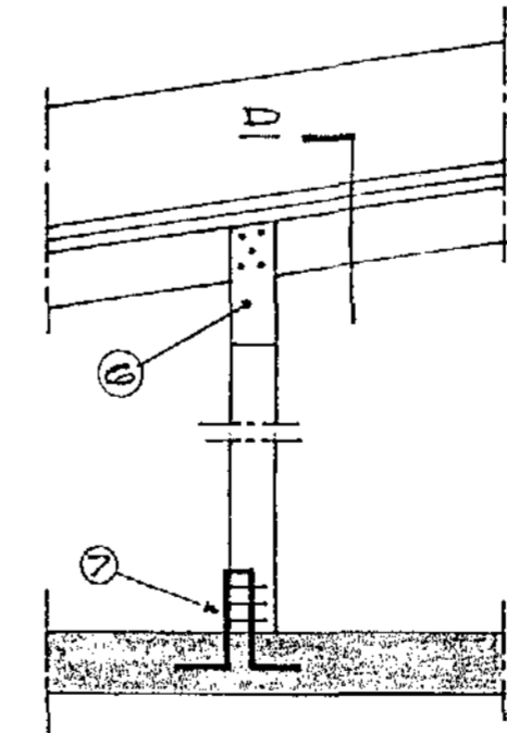
SKURÐUR C, M.182
