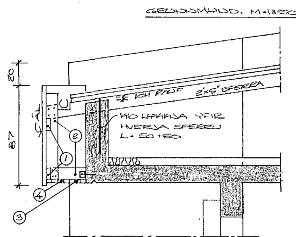
SKURÐUR B, M.182
