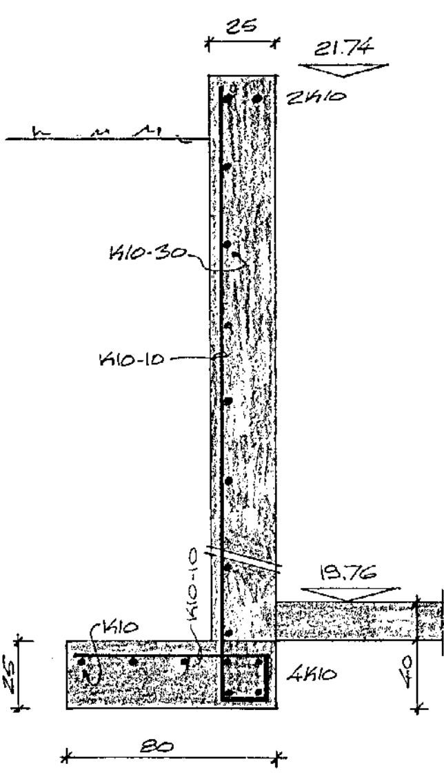
SAÐJÆÐUR 3. M. 1:20
