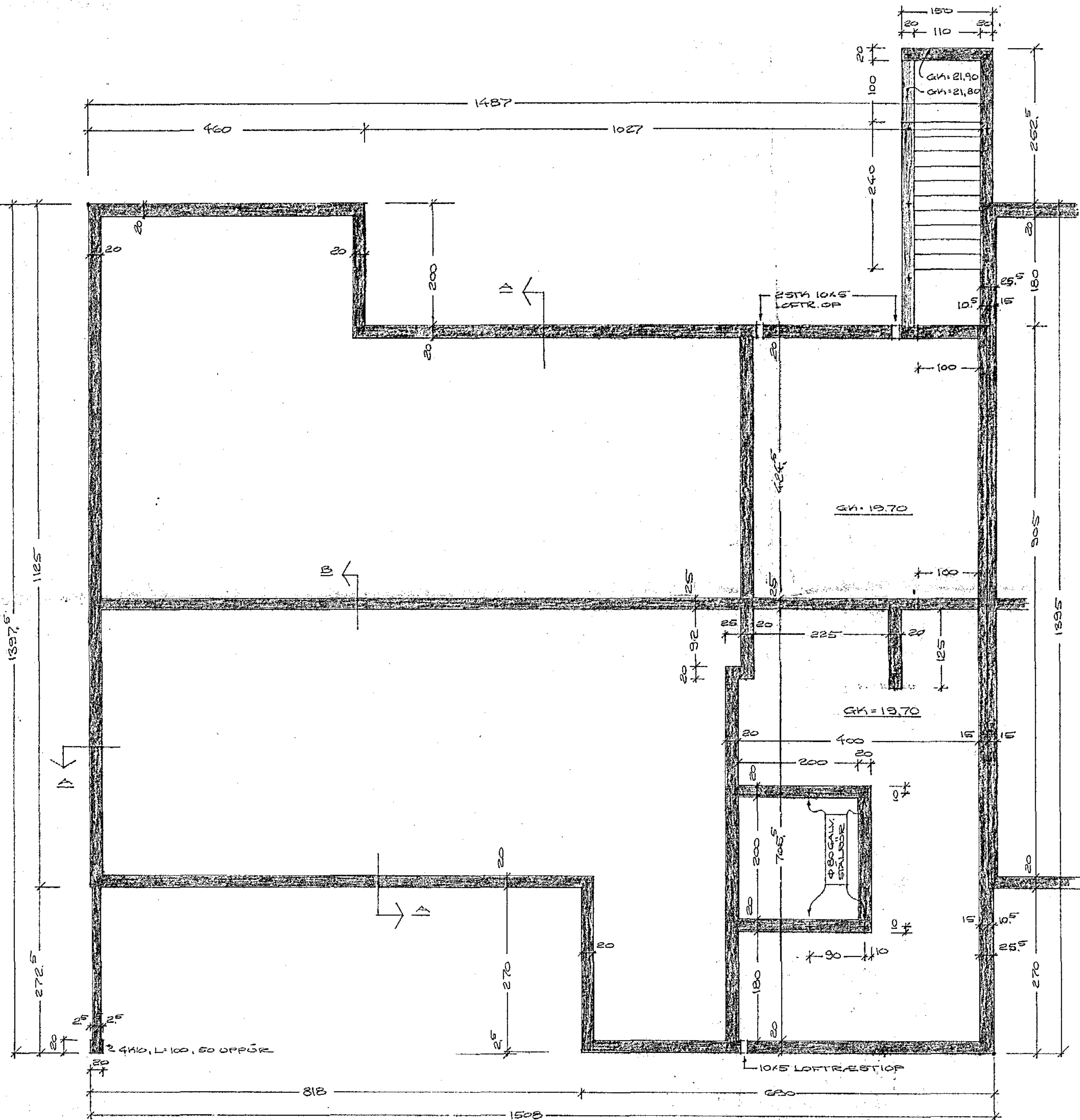
GRUNNMYND, M=1:50
