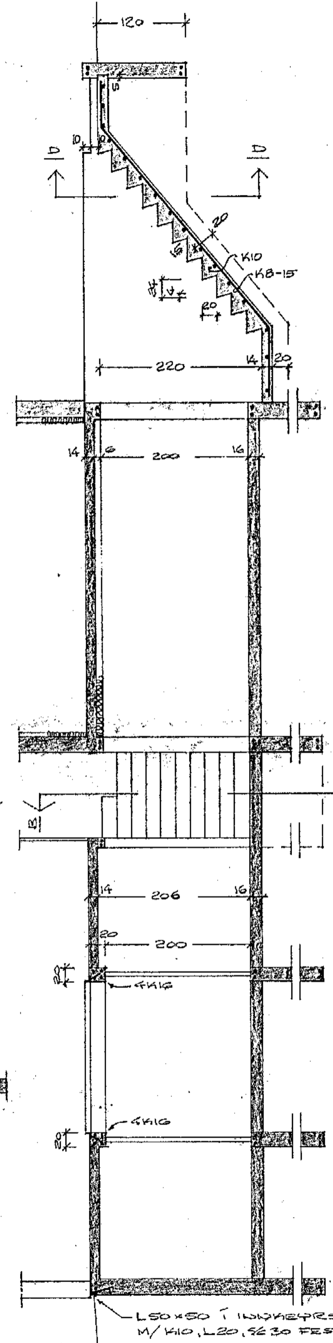
SKURÐUR A-A, M=1:50
