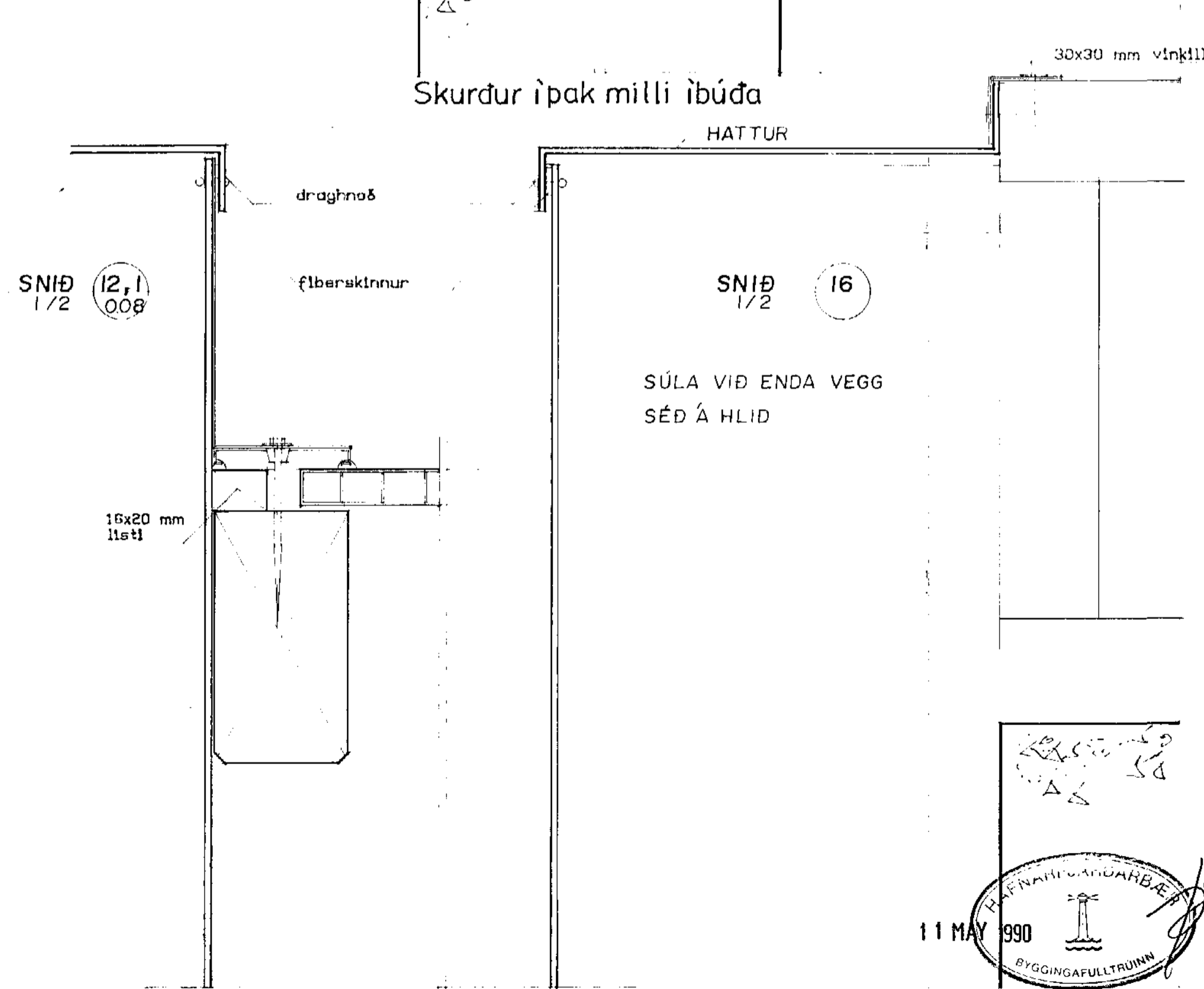
Skurdir í súlur
