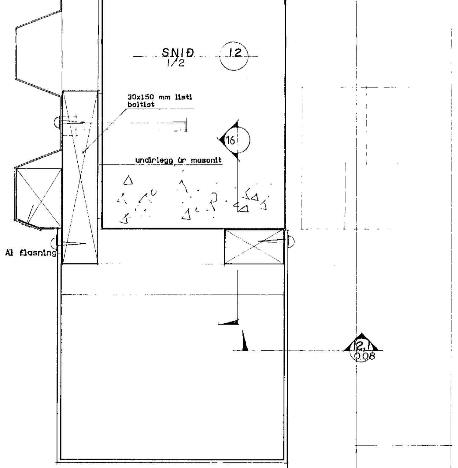
Lárættur skurður í endavegg fyrir ofan pak
