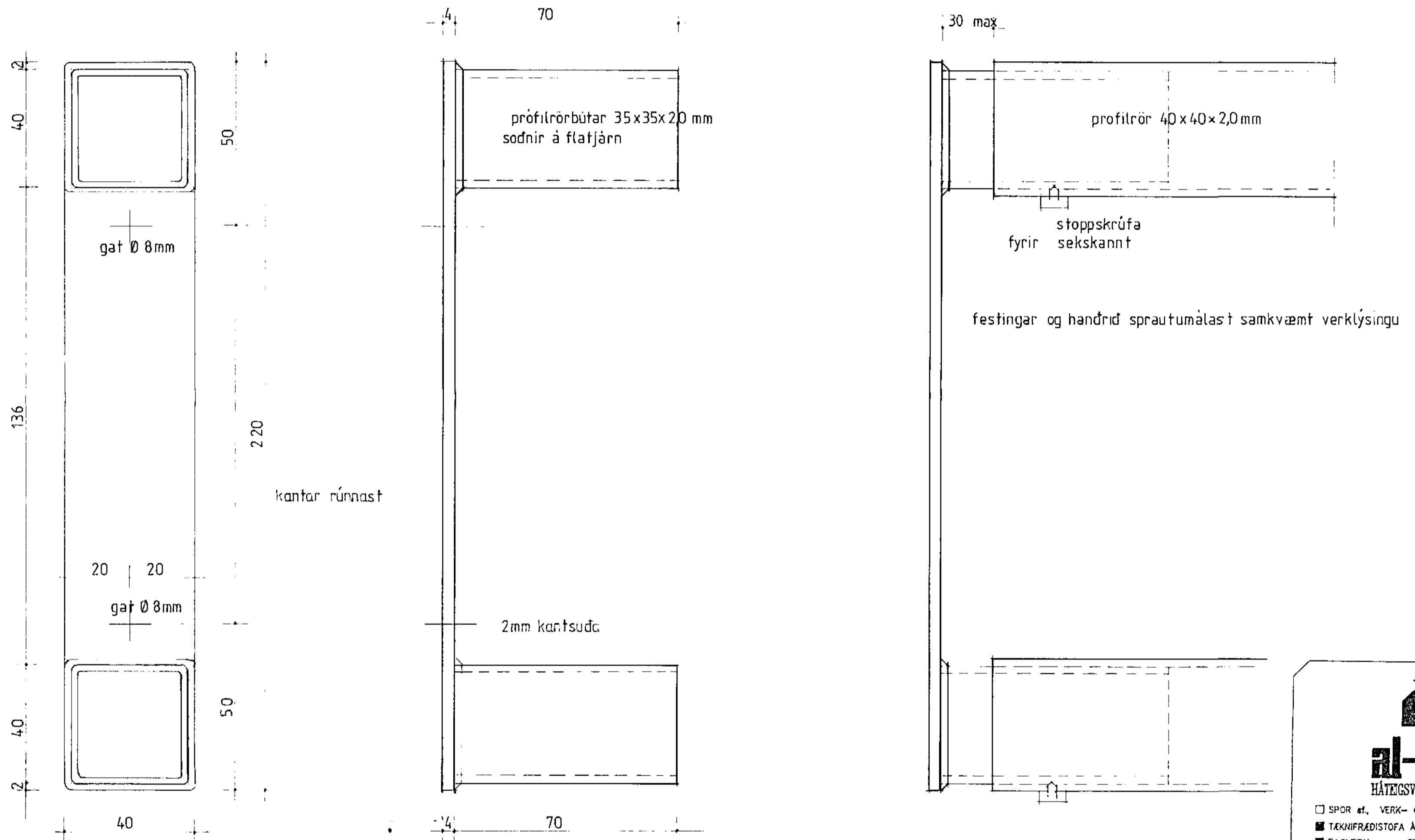
Handriðsfesting 1:1
