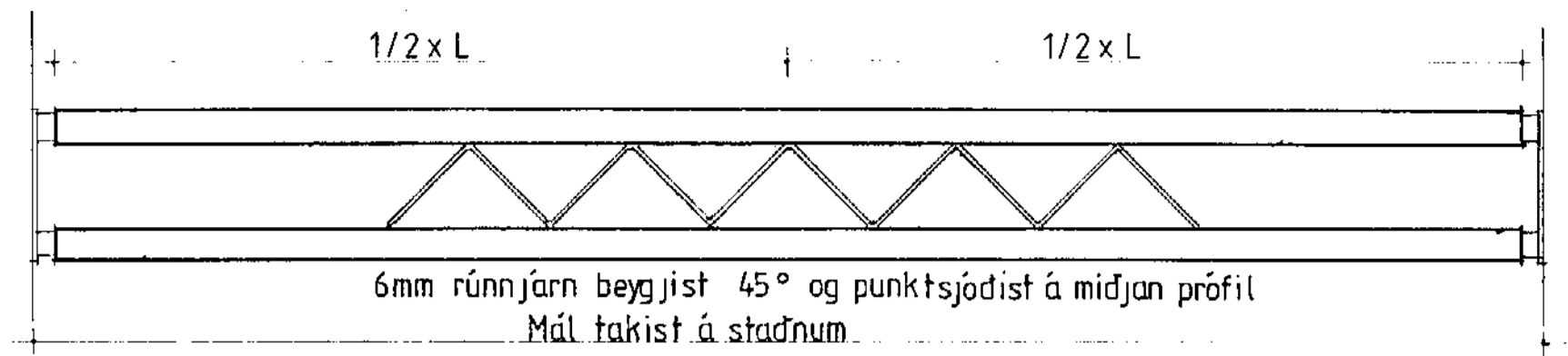
Handrið 1:20
