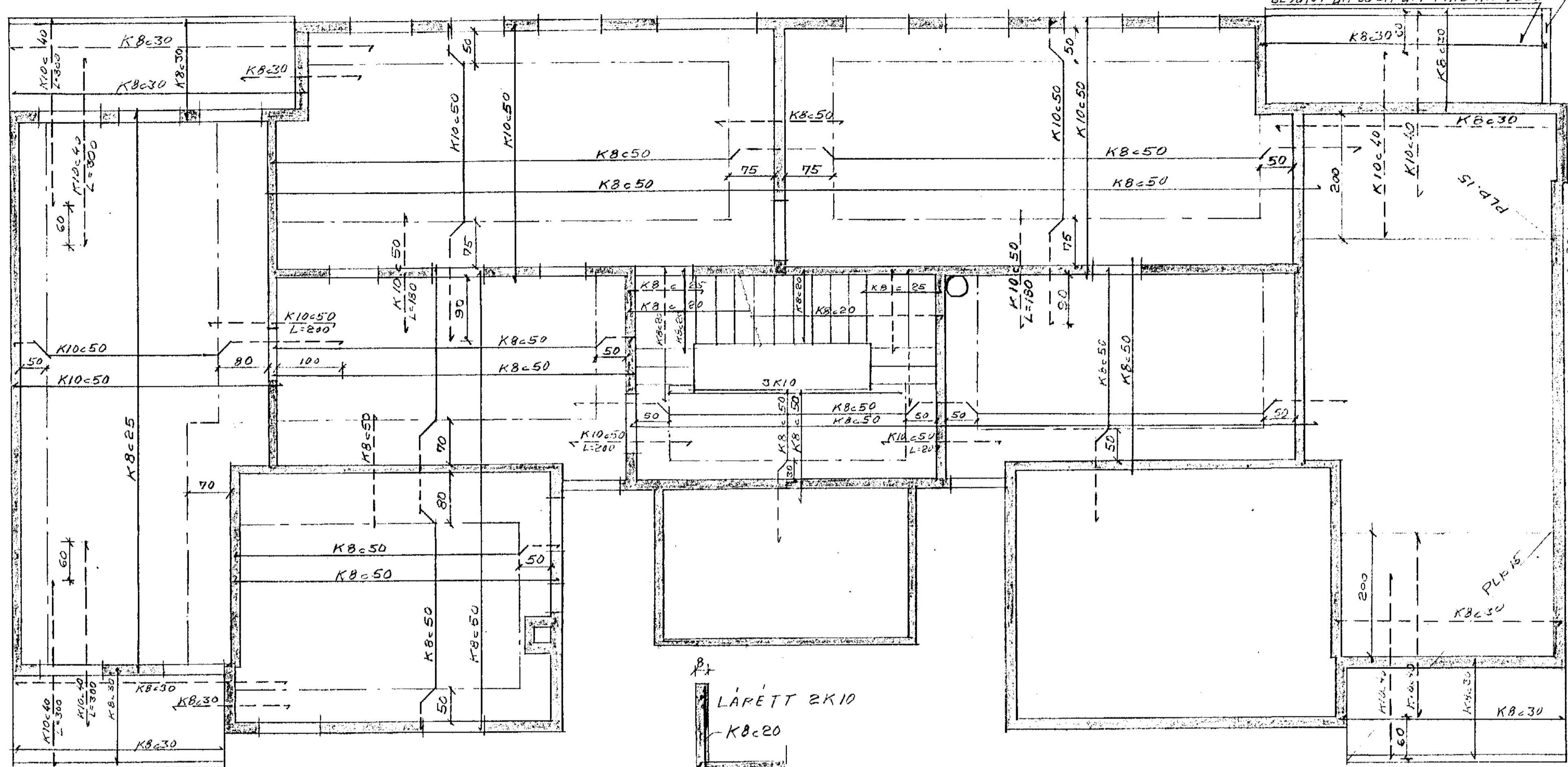
PLATA YFIR KJALLARA PLOTUR 15CM
