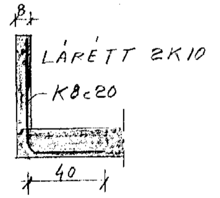
SNID Í SVALHANDRÍÐ
