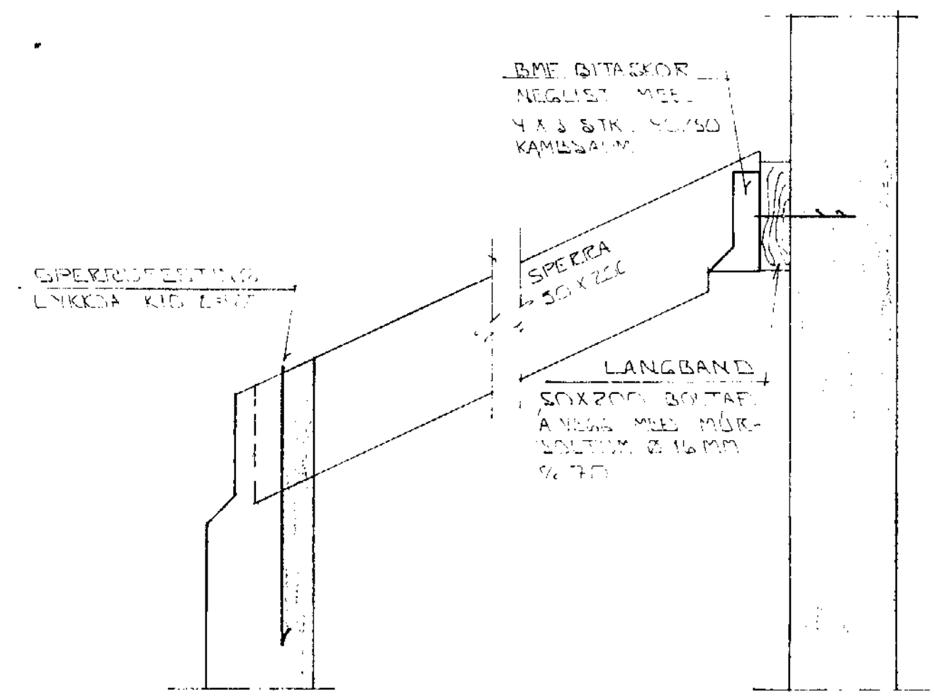
SNIÐ 5-5 1:10
