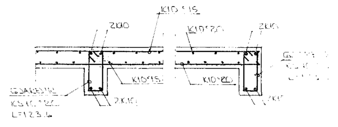
SNID D - D 1:20
