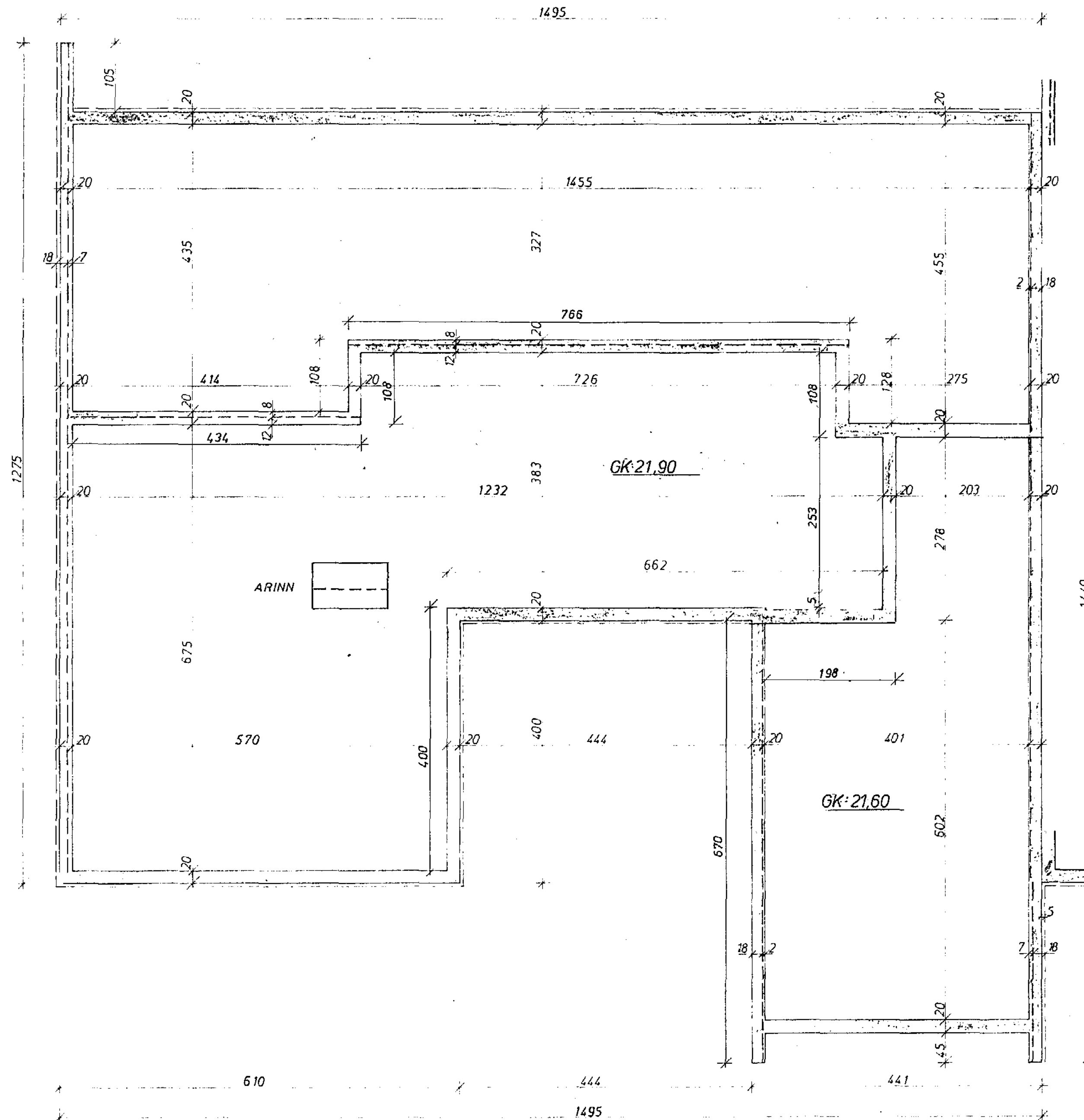
GRUNNMYND 1:50
