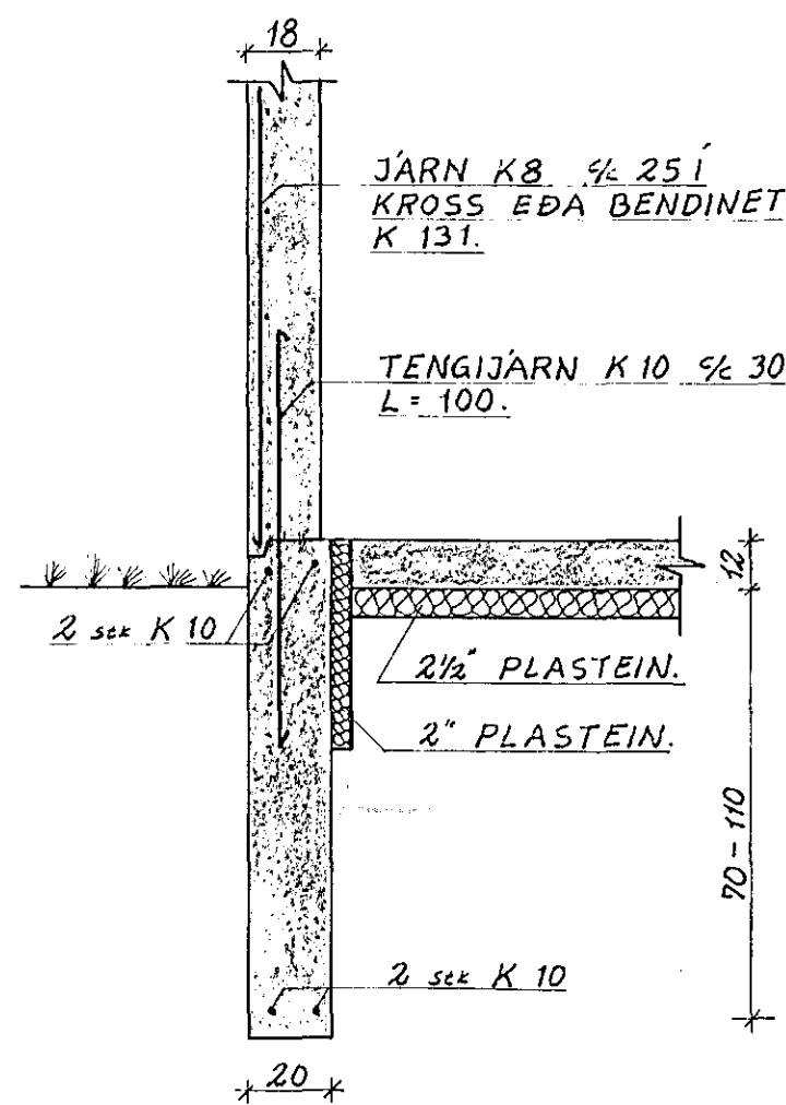
SNID D-D 1:20
