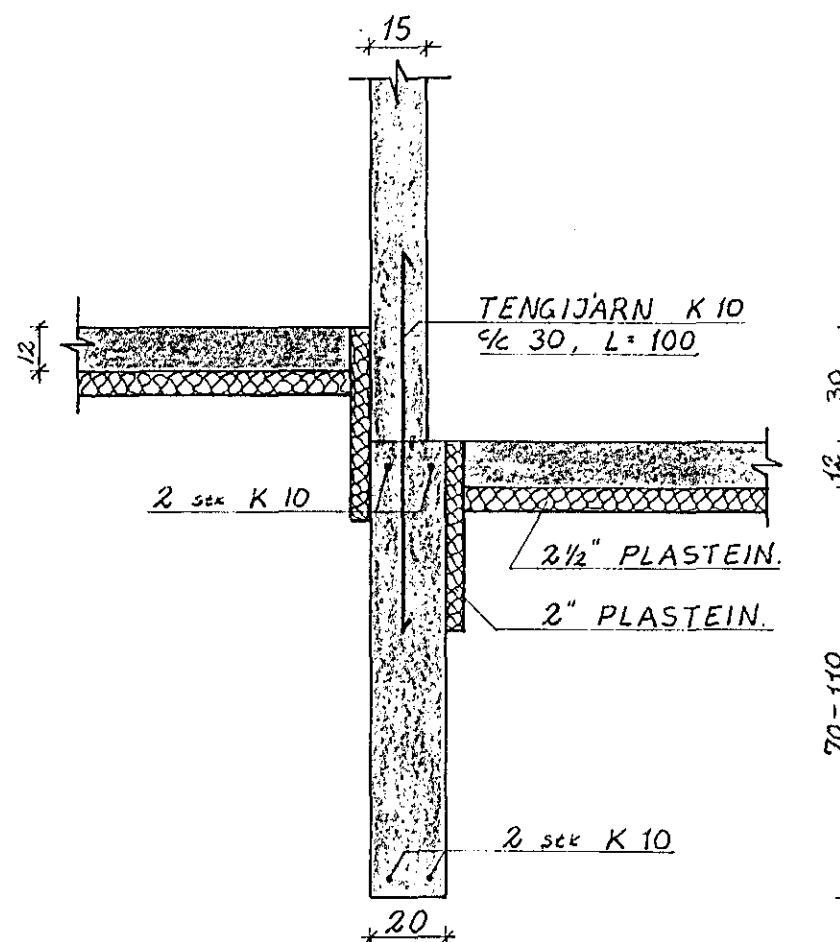
SNID D-D 1:20
