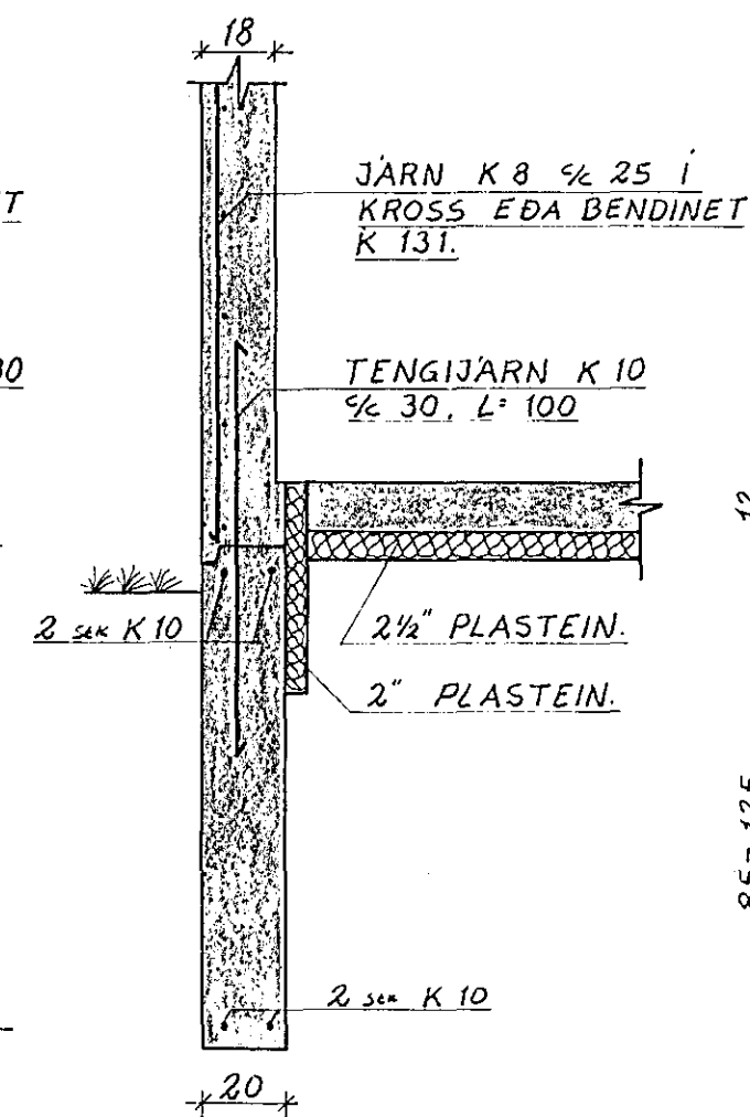
SNID B-B 1:20
