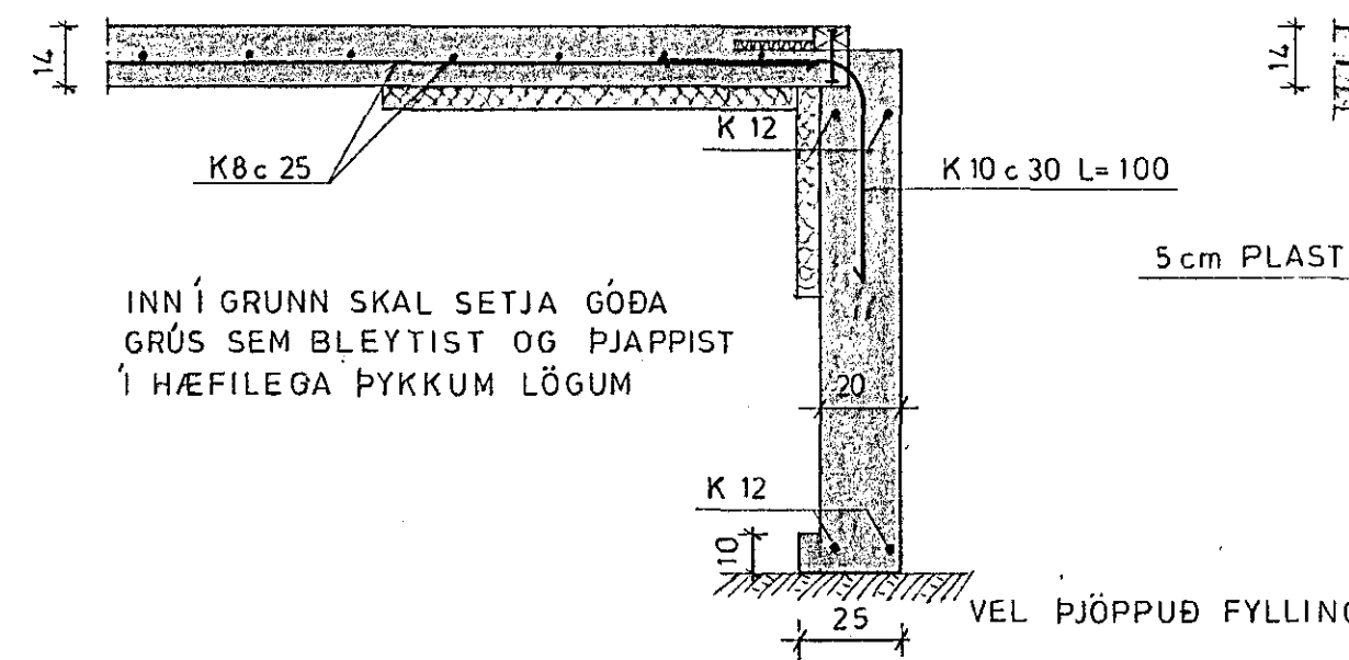
SNID A-A 1:20
