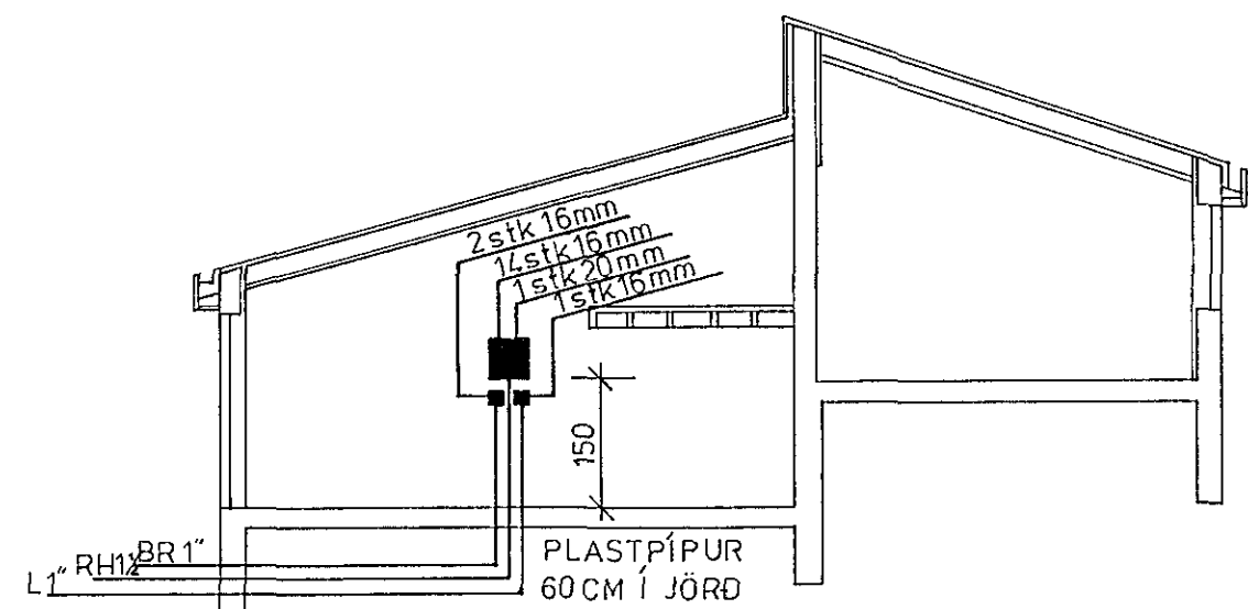
SNEIÐING 1:100
