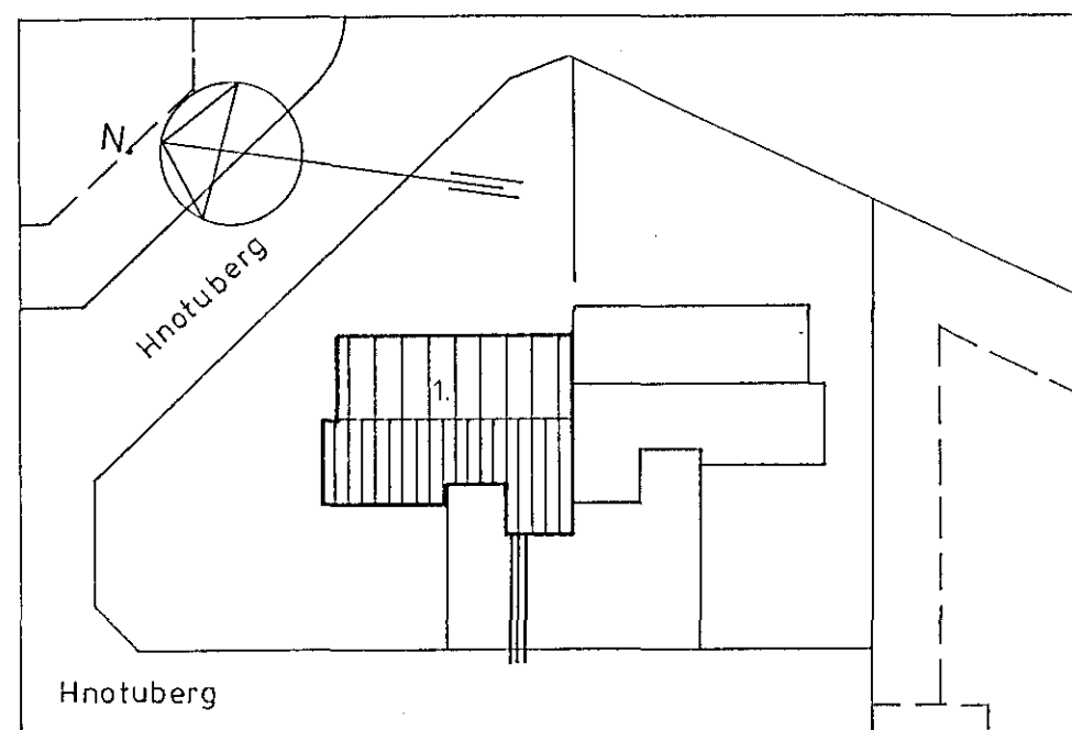
AFSTÖÐUMYND 1:500
