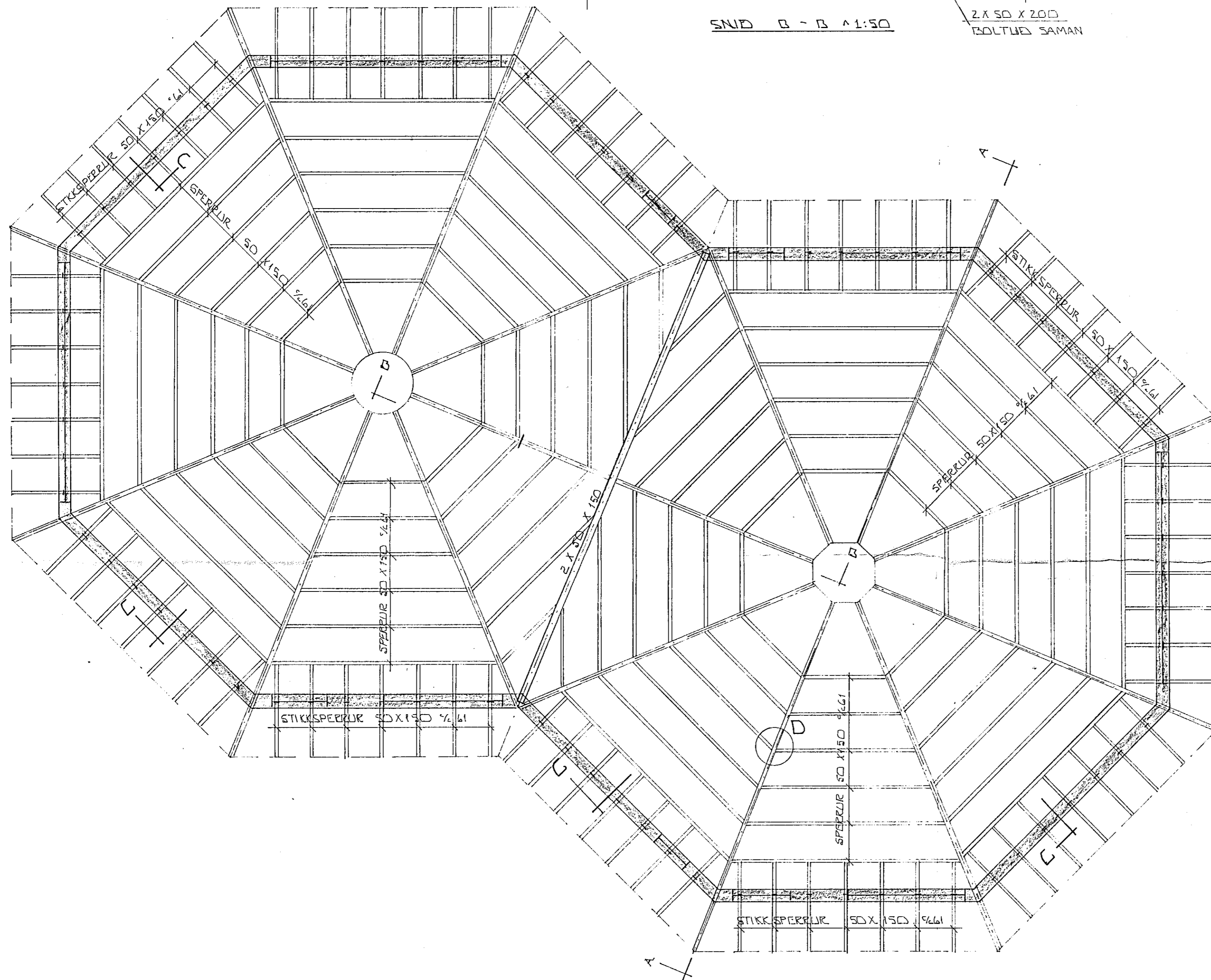
GRUNNMYND ÞAKVIRKIS 1:50
