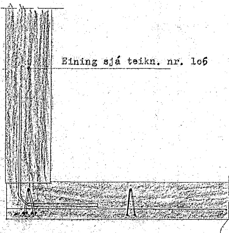
Snið A-A M=1:10
