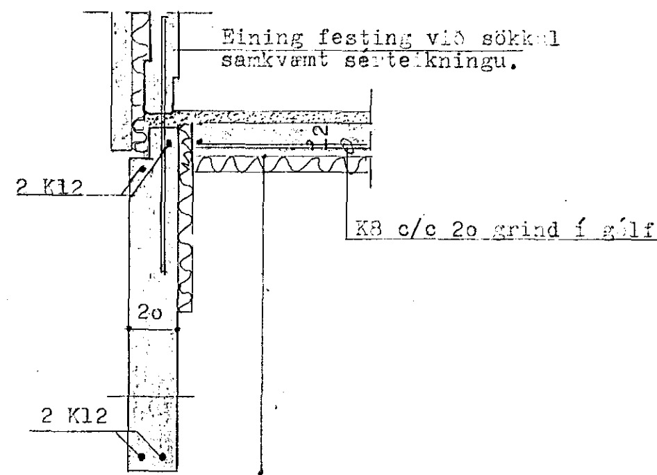
SNID A-A, M=1:20
