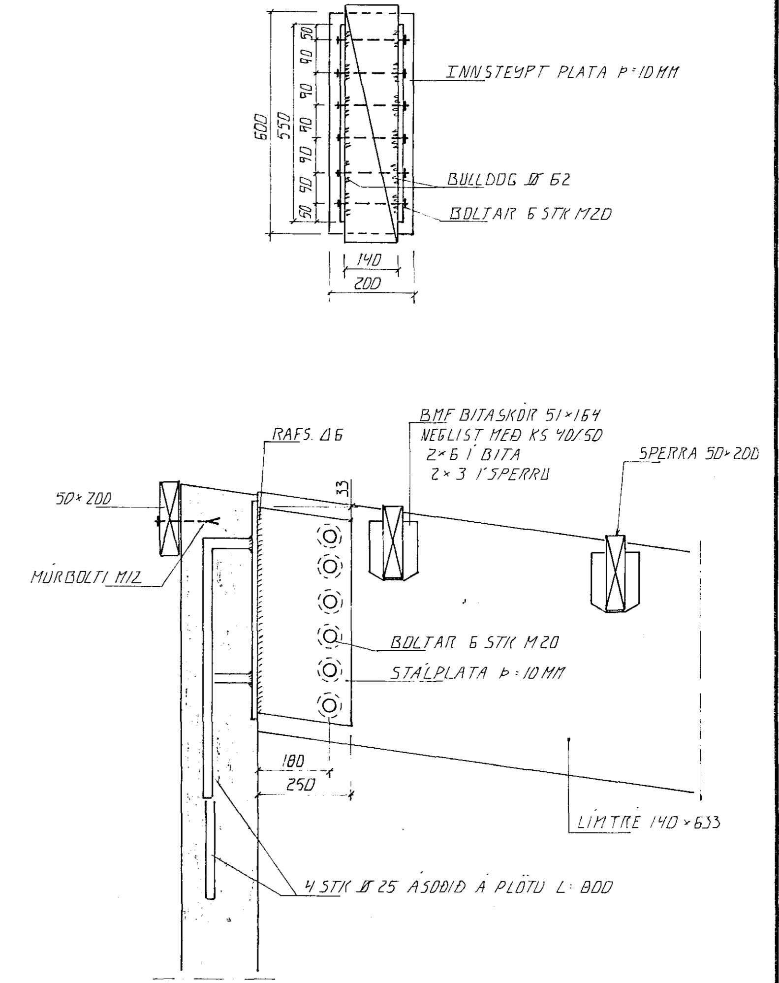
LÍMTRÉSBITI VID VEGG, 1:10
