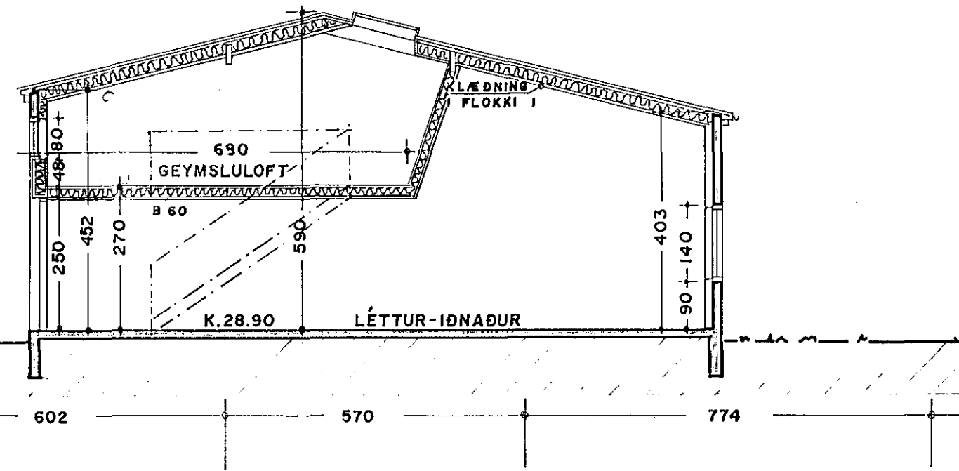
SNEIÐING. C-C
