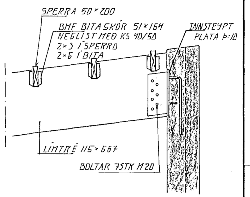
LÍMTRÉ VIÐ VEGG. 1:20
