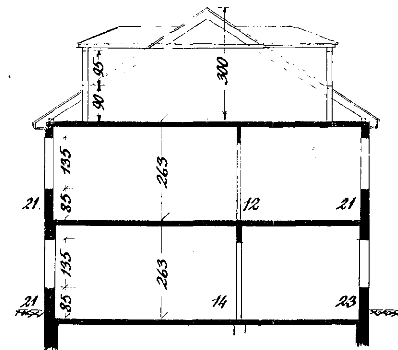
þverskurður
