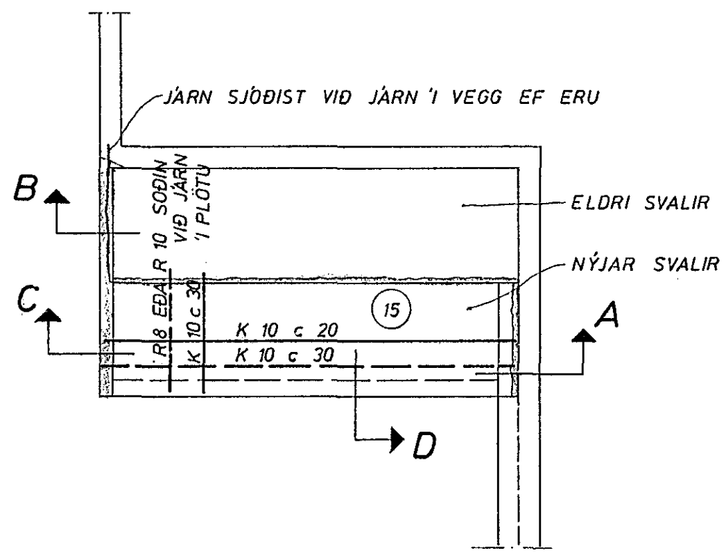
GRUNNMYND 1: 50
