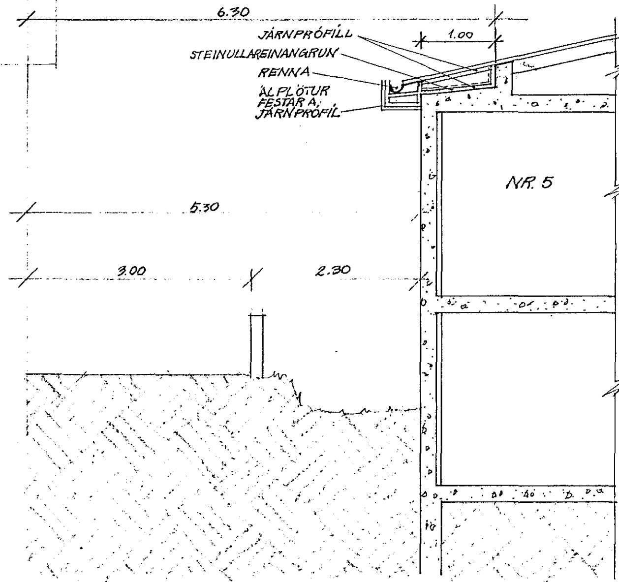
SNEIÐING AF BRUNAVEGG M. 1:50
