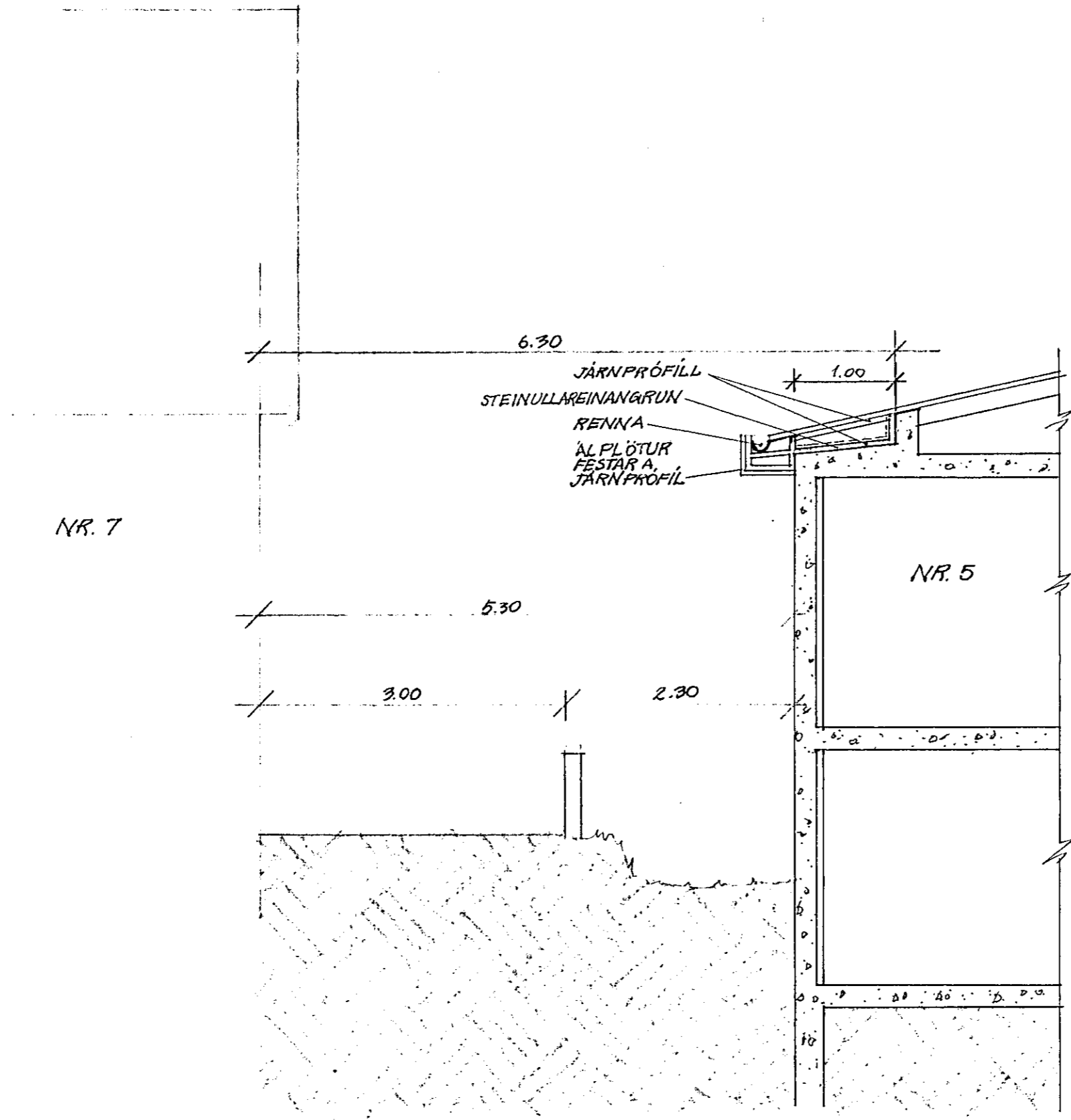
SNEIÐING AF BRUNAVEGG M. 1:50
