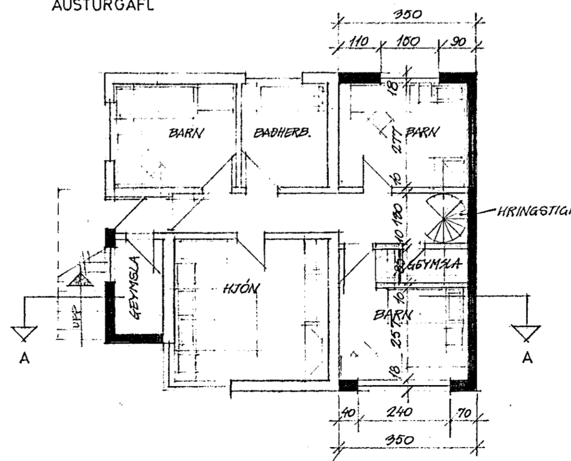
AUSTURGAFL
