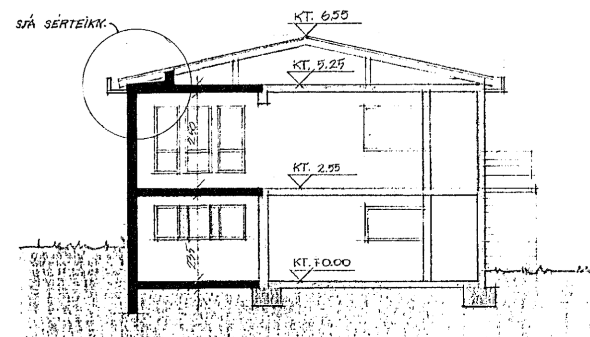
NORDURHLIÐ
