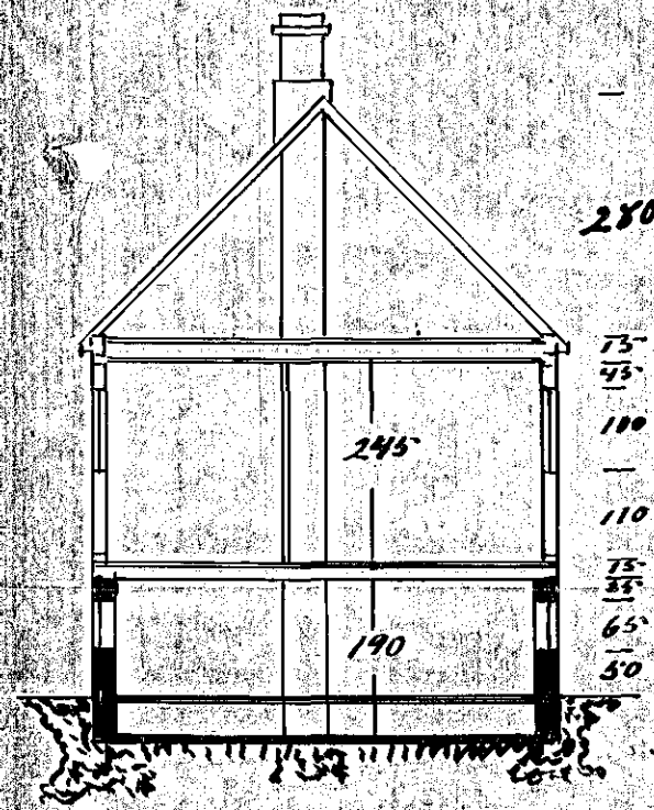
Þverskurður
