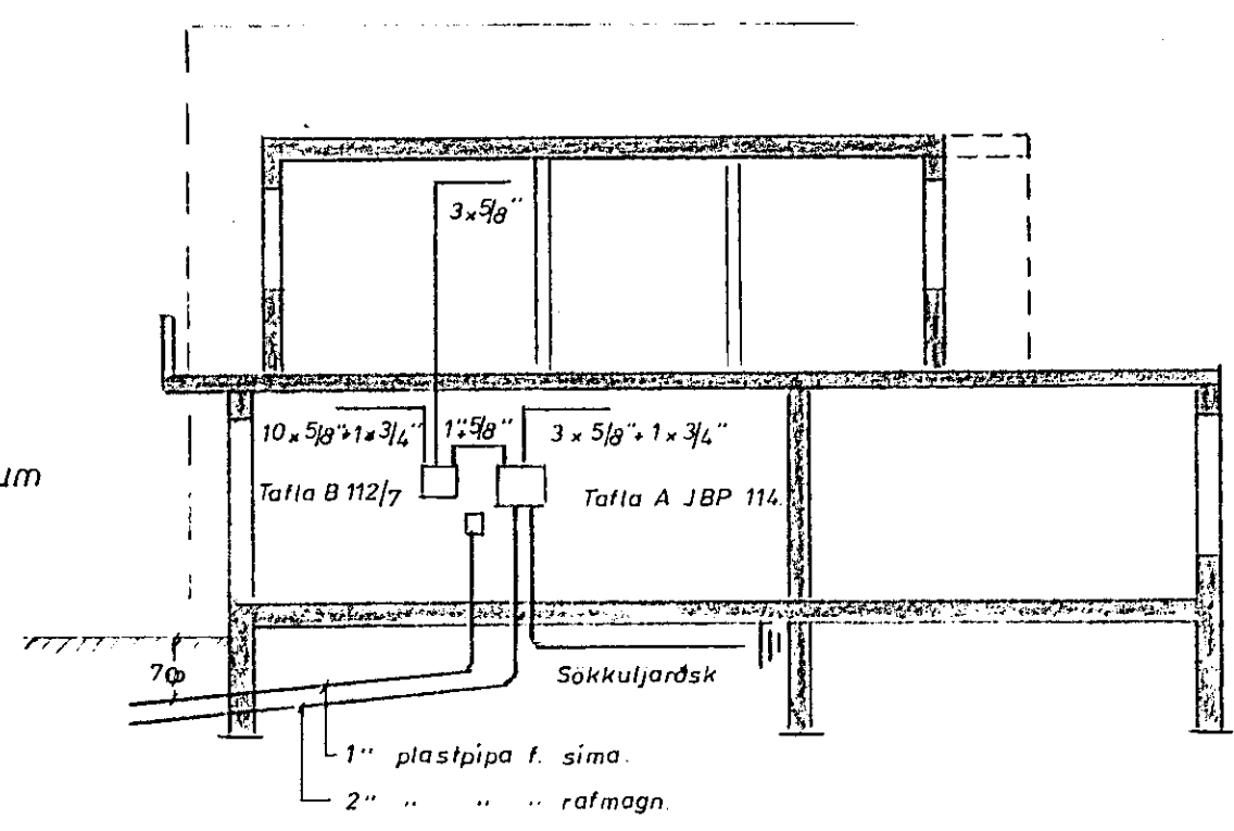
Skurður A-A M: 1:100.
