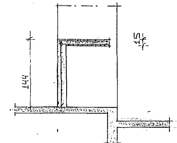
JARNAGRIND I MIDJUM VEGGI K8%25# LÖBRET JARN I=320 SNID A-A 1:50
