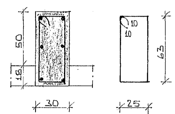
SNID I SÚLU S2 1:20
