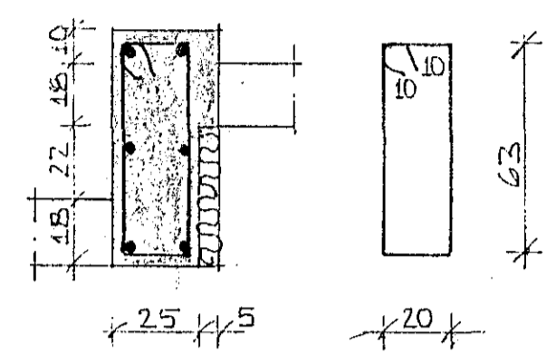
SNID I SÚLU S1 1:20
