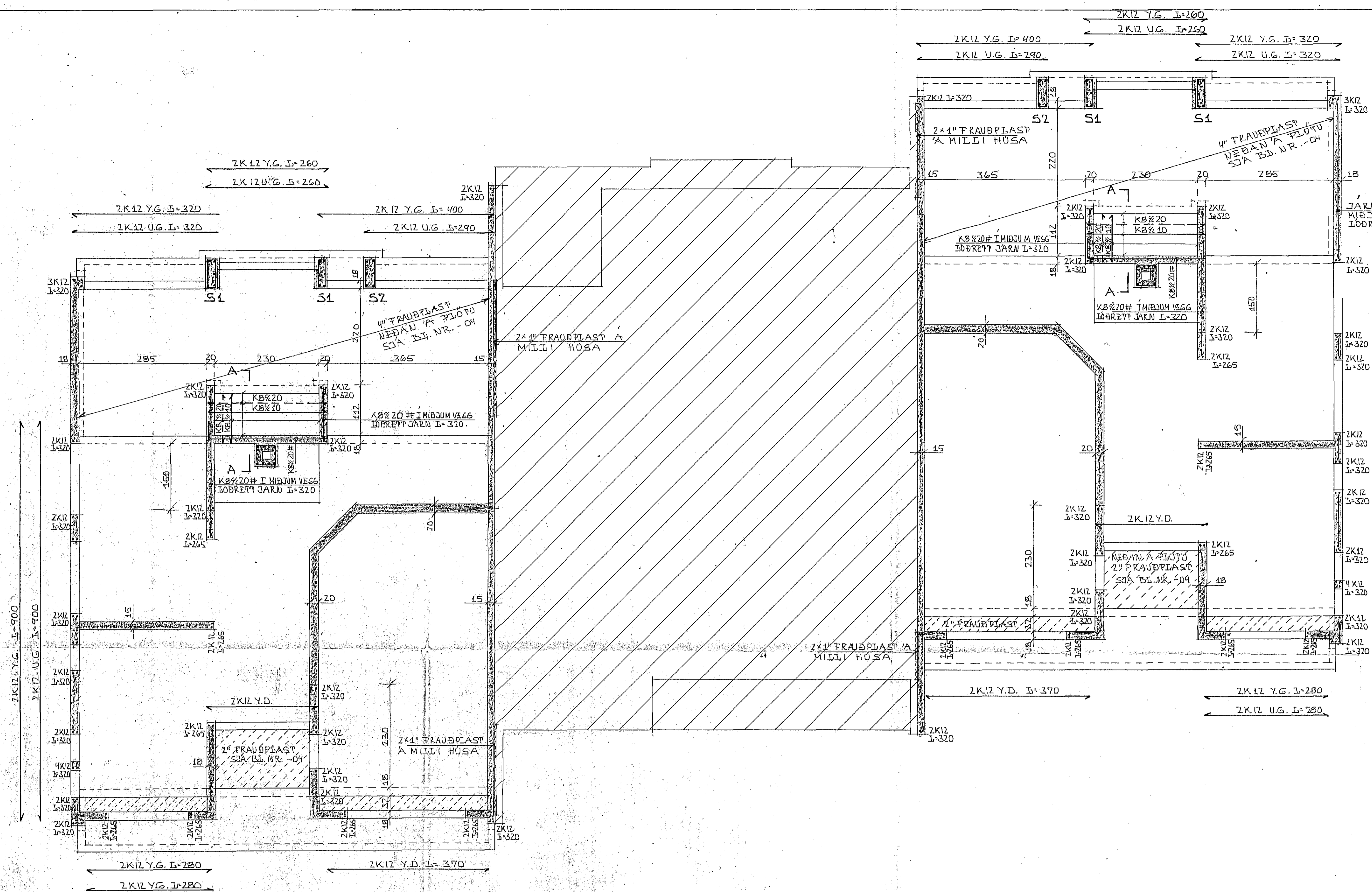
GRUNNMYND 1:50
