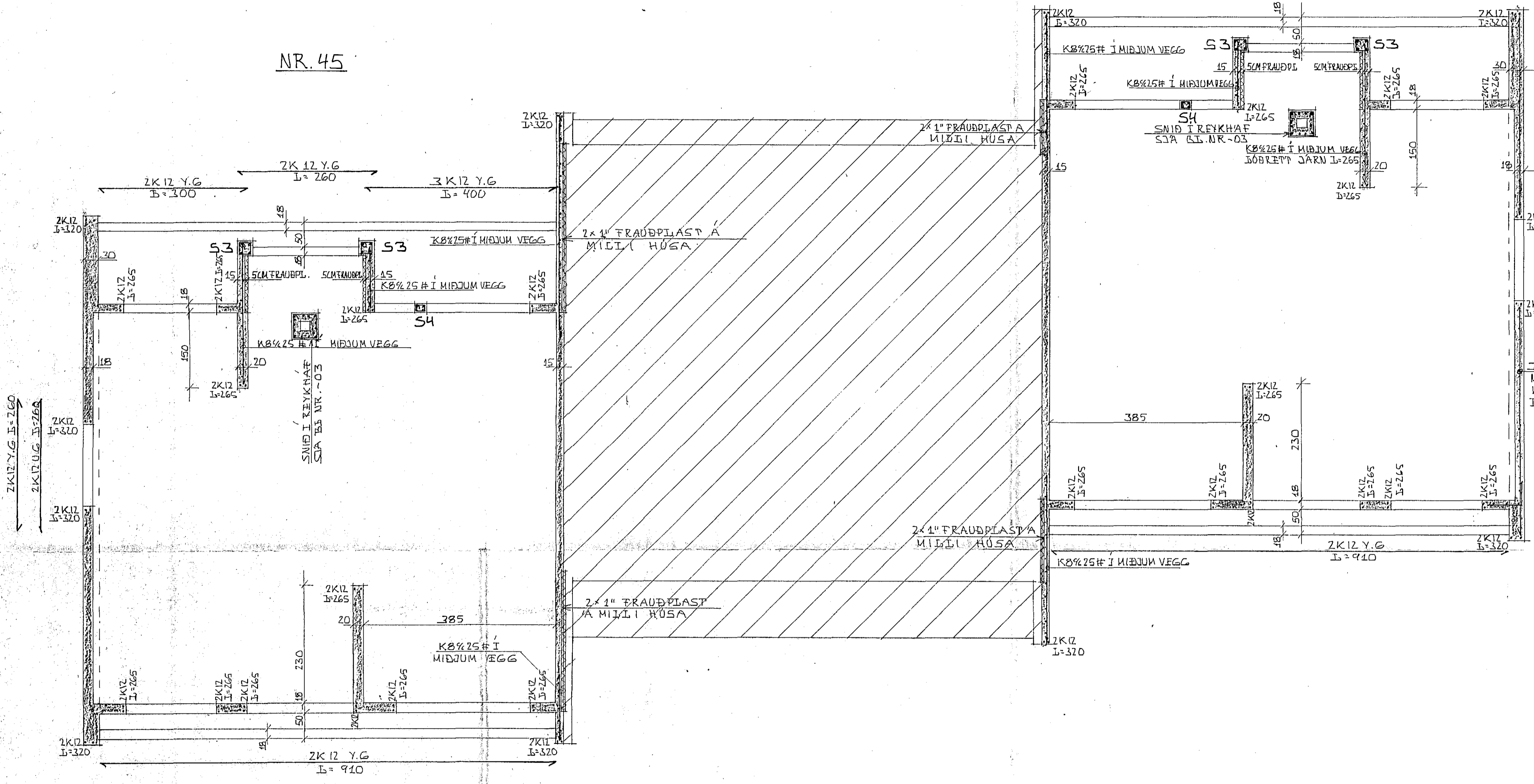
GRUNNMYND 1:50
