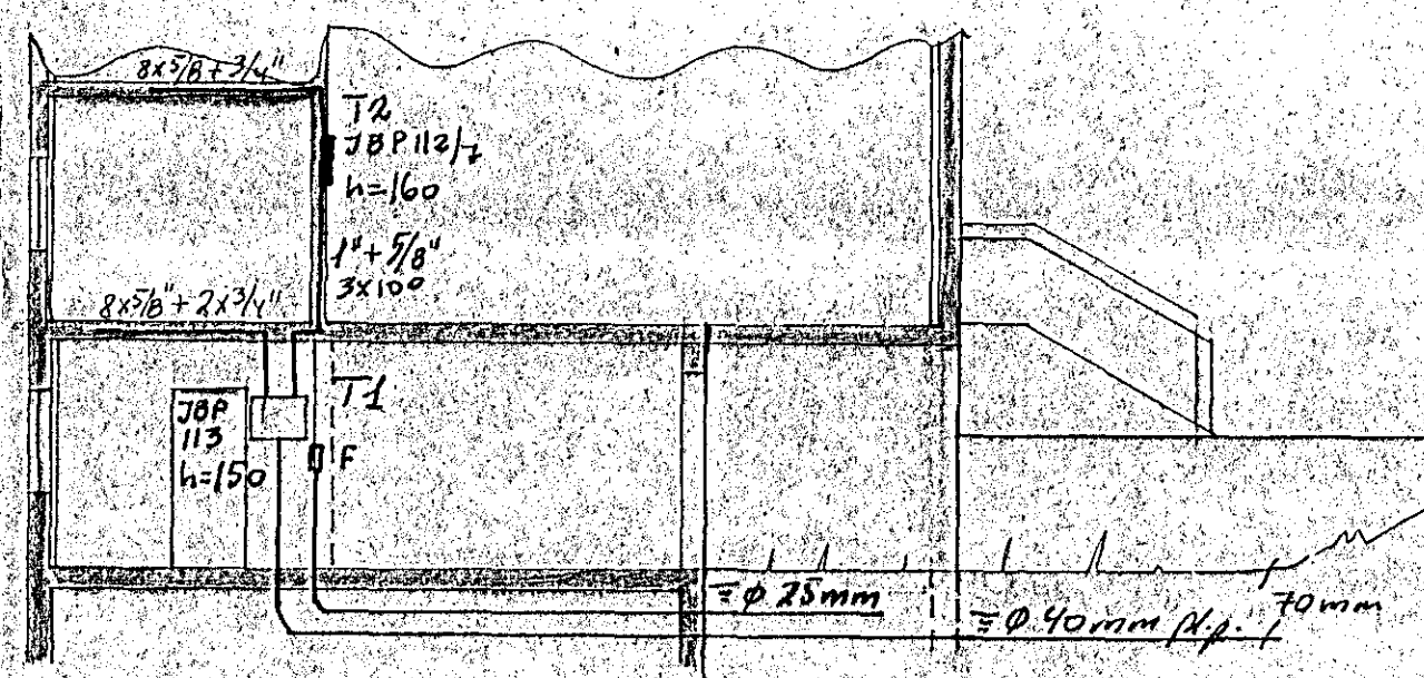
SNID A-A Í INNTAK M 1:100
