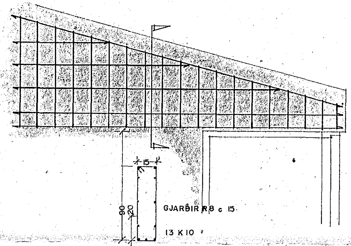
BITI 4. M. 1:20
