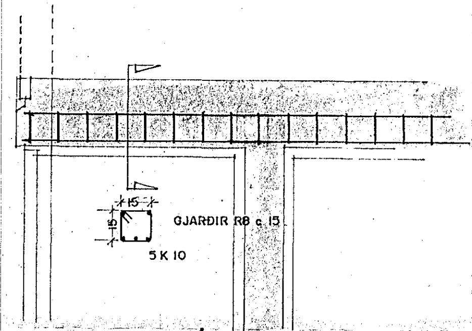
BITAR YFIR HORNGLUGGUM Í STOFU M. 1:20
