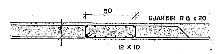
BITI 4. M. 1:20
