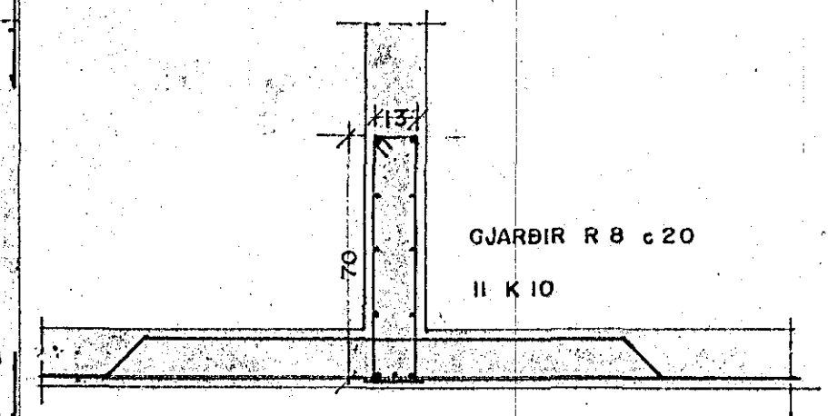
BITI 6. M. 1:20
