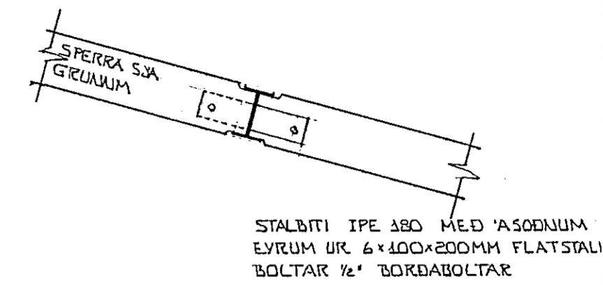
SNID C-C 1:20 AF TEIKN. NR. 08
