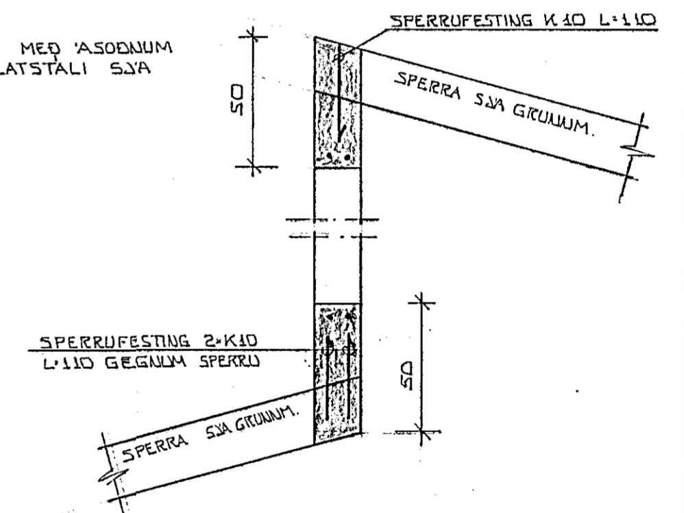
SNID E-E 1:20 AF TEIKN. NR. 06
