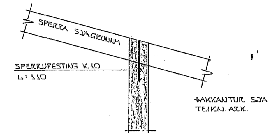
SNID D-D 1:20 AF TEIKN. NR. 06
