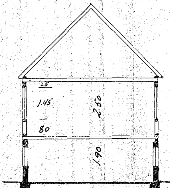
Skurður
