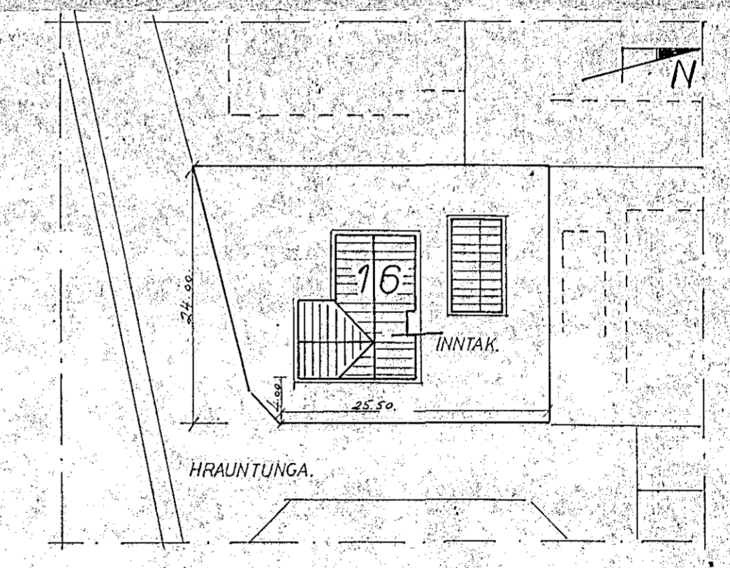
AFSTÖÐUMYND 1:500
