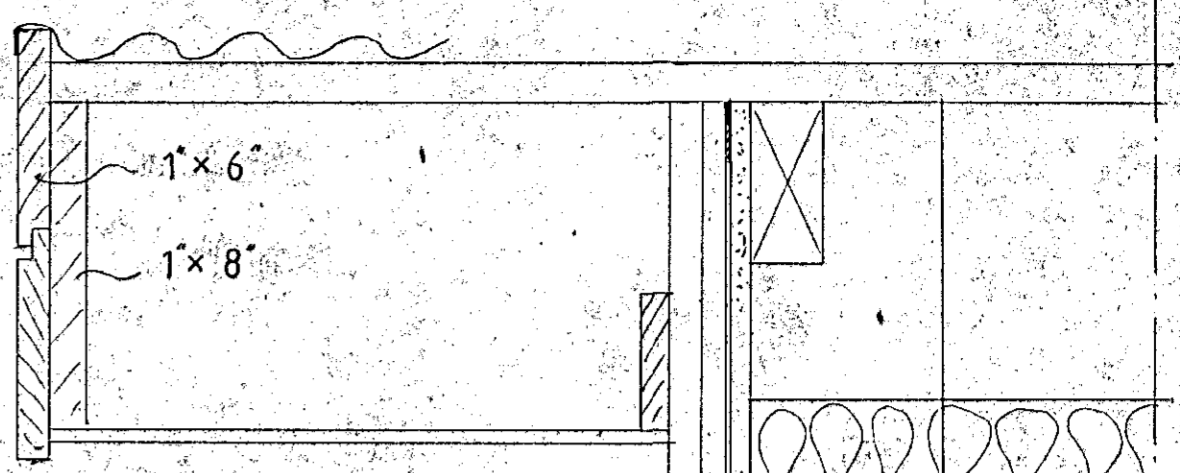
LÓÐRÉTT SNIÐ Í STAFN
