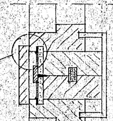
LÁRÉTT SNIÐ - SAMSETN. EININGA
