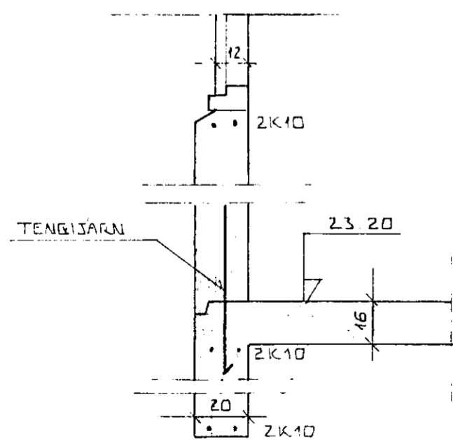
SNID D Í SÚLU S2 1:20
