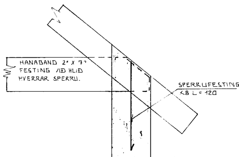
SÉRMYND II 1:10
