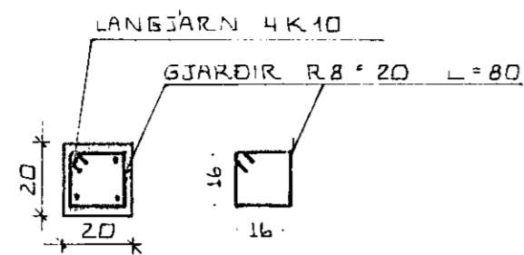
SÚLA S1 1:20
