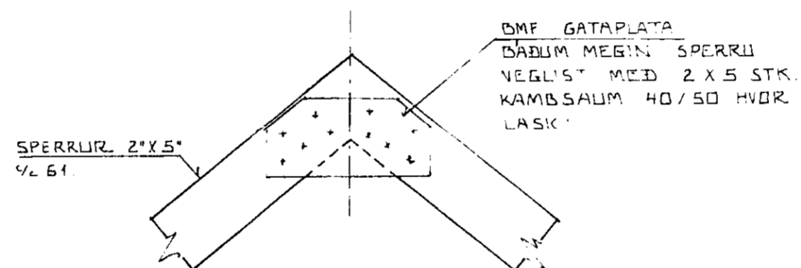
SÉRMYND I 1:10
