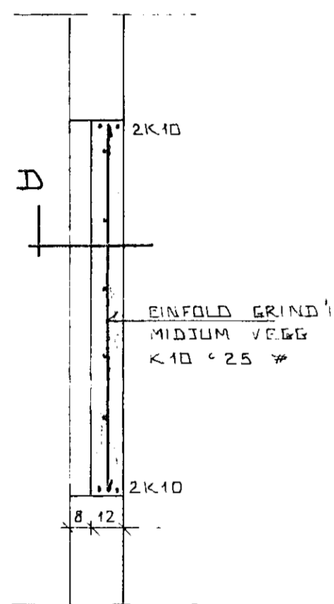
SÚLA S2 1:20
