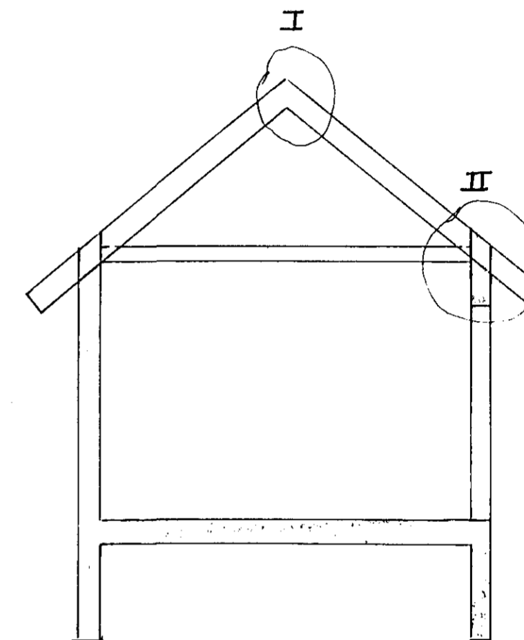
SNID B-B 1:50
