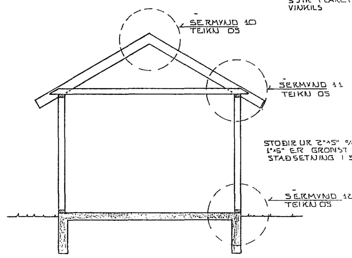
SNID B-B 1:50
