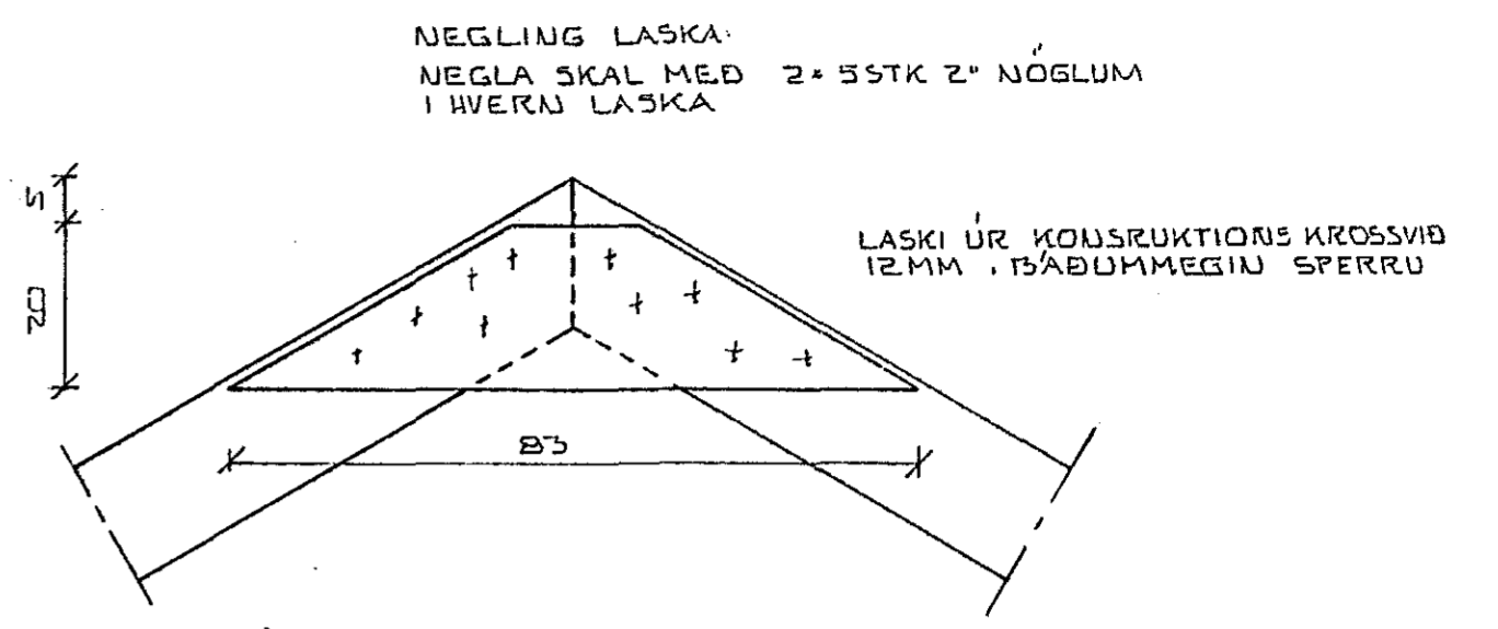
SERMYND 10 1:10
