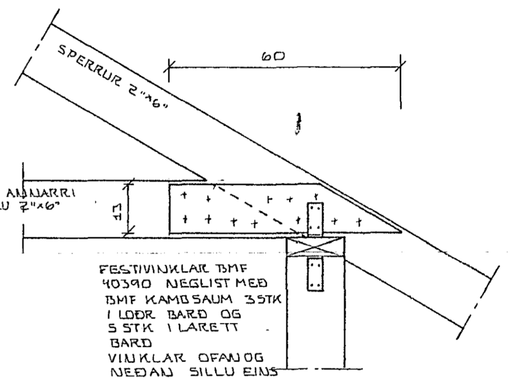
SERMYND 11 1:10
