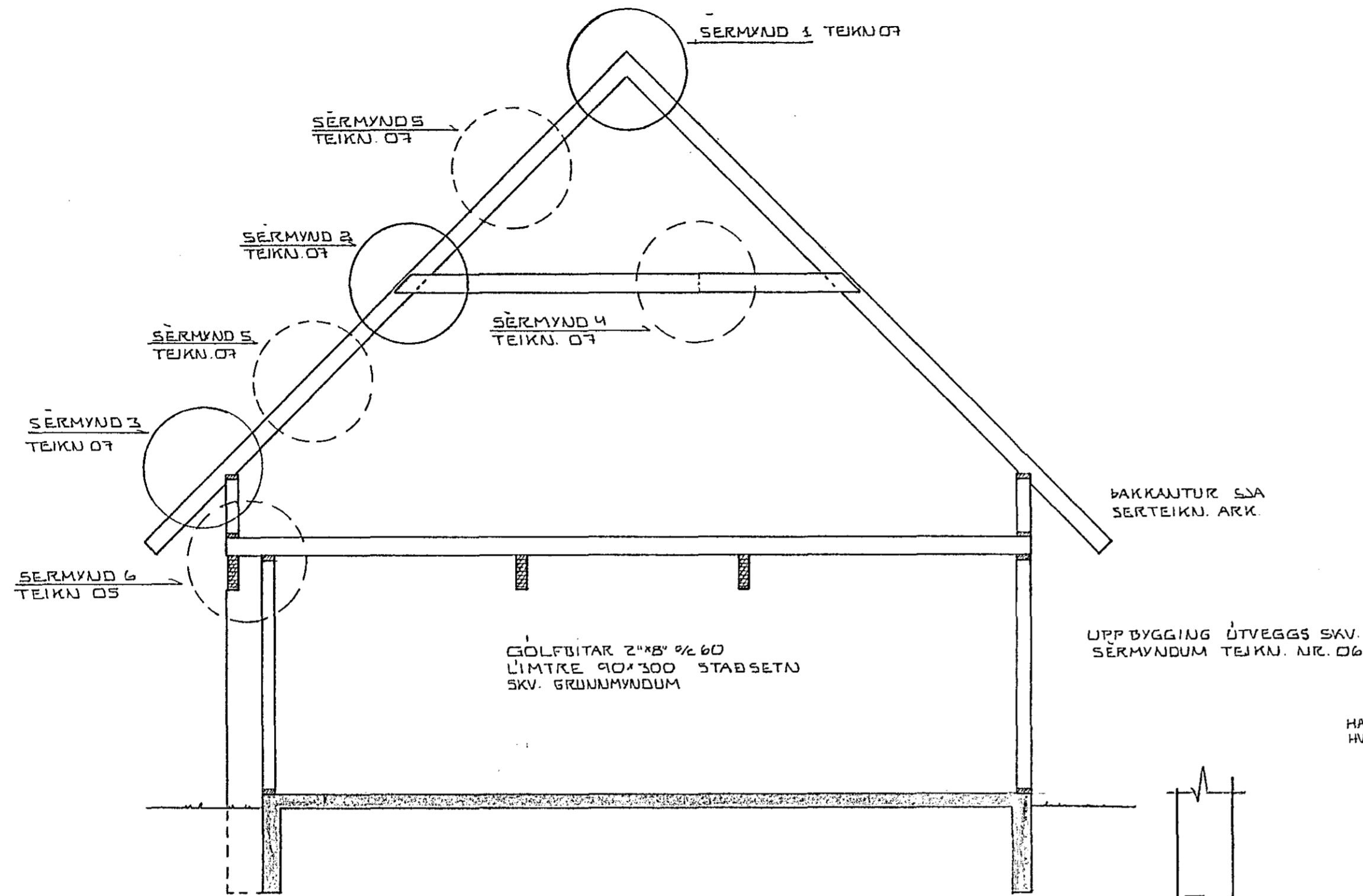
SNID A-A 1:50
