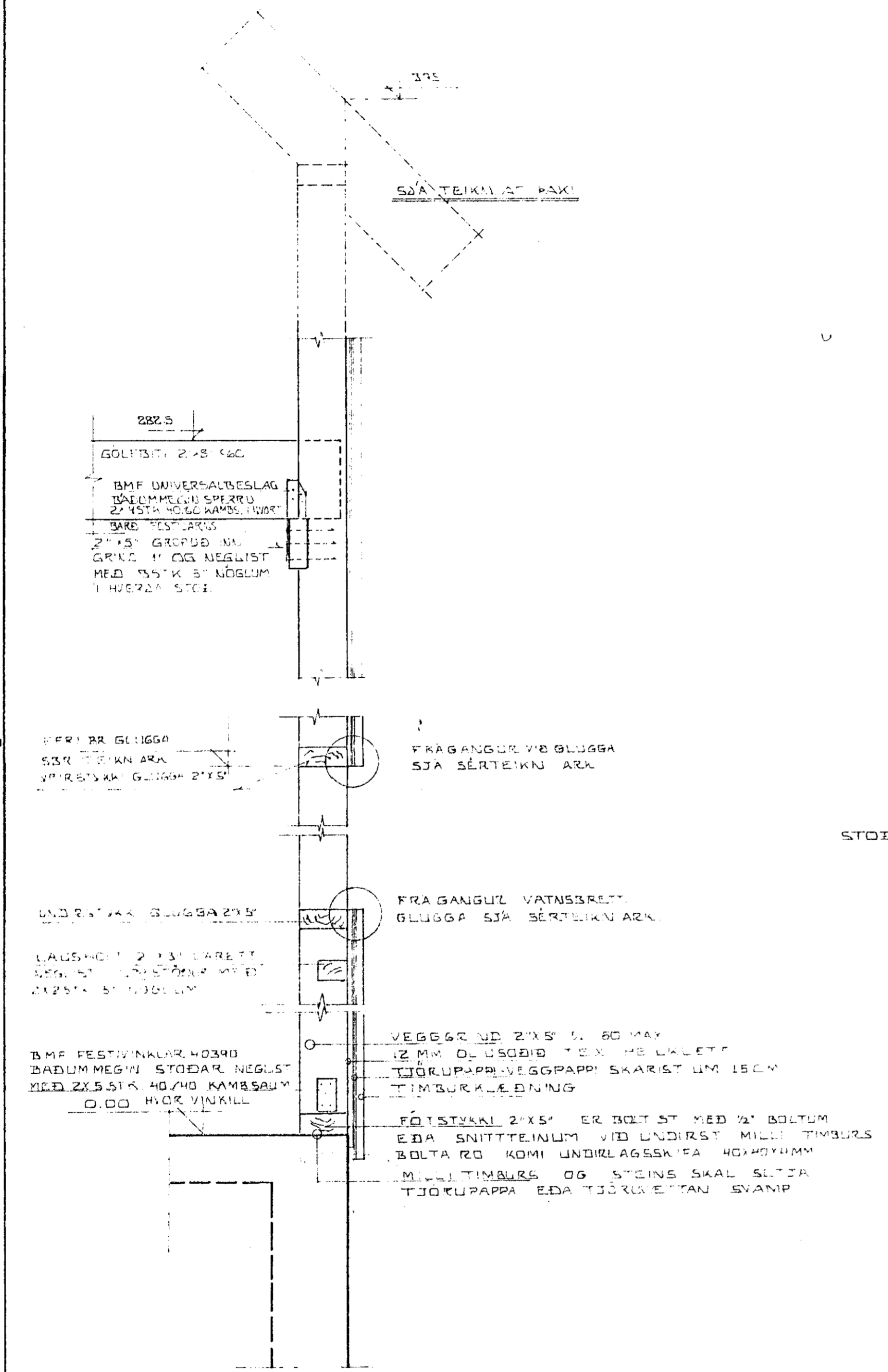
SNIÐ Í ÚTVEGG MEÐ GLUGGA 1:10
