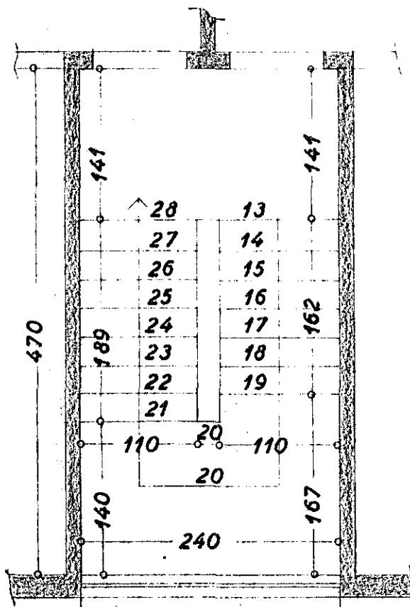
Grunnmynd af I. hæð á II.
