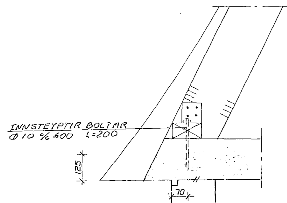
SNID Í FESTINGAR BAKS M 1:10
