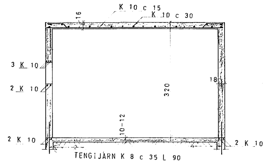
SNID A-A 1:50
