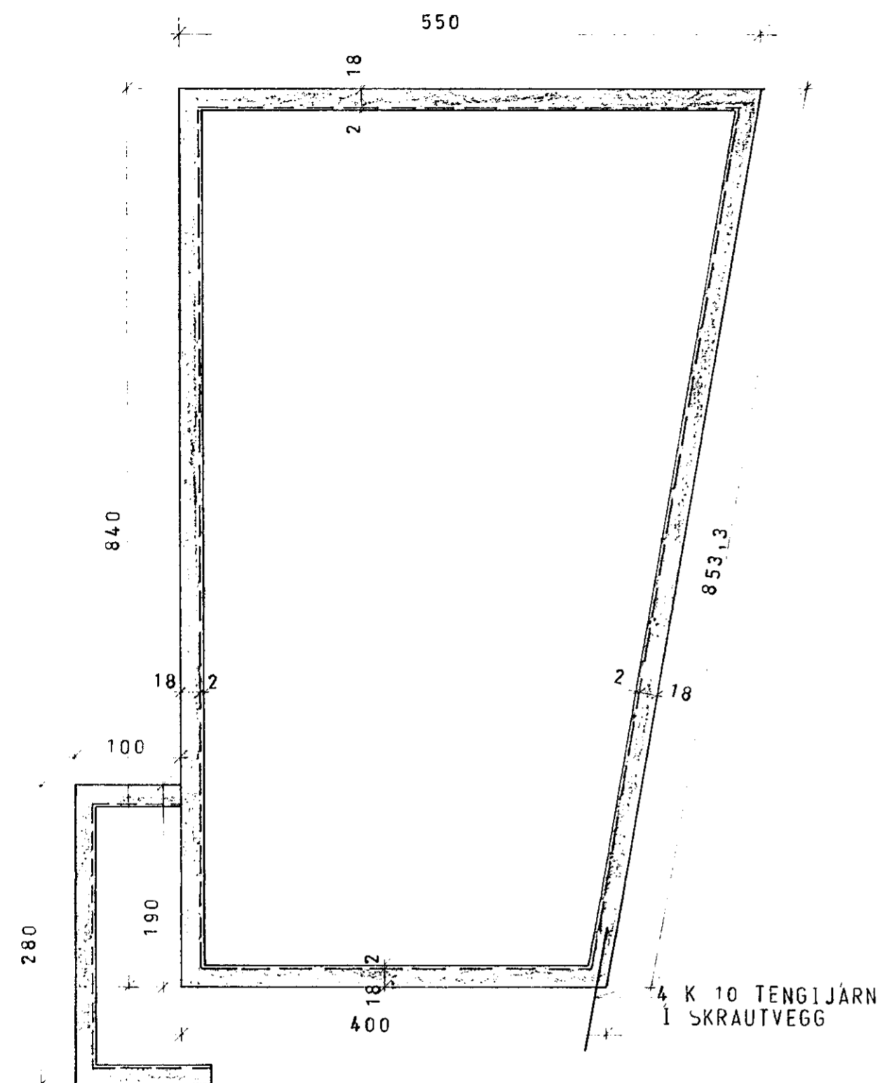
UNDIRSTÖÐUR 1:50
