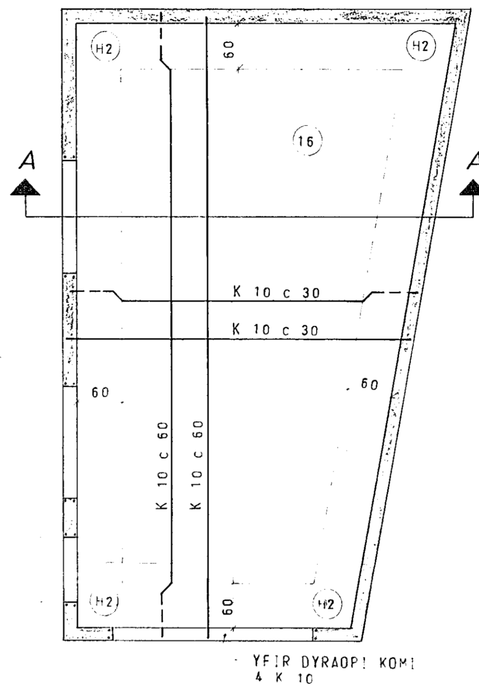
GRUNNMYND 1:50
