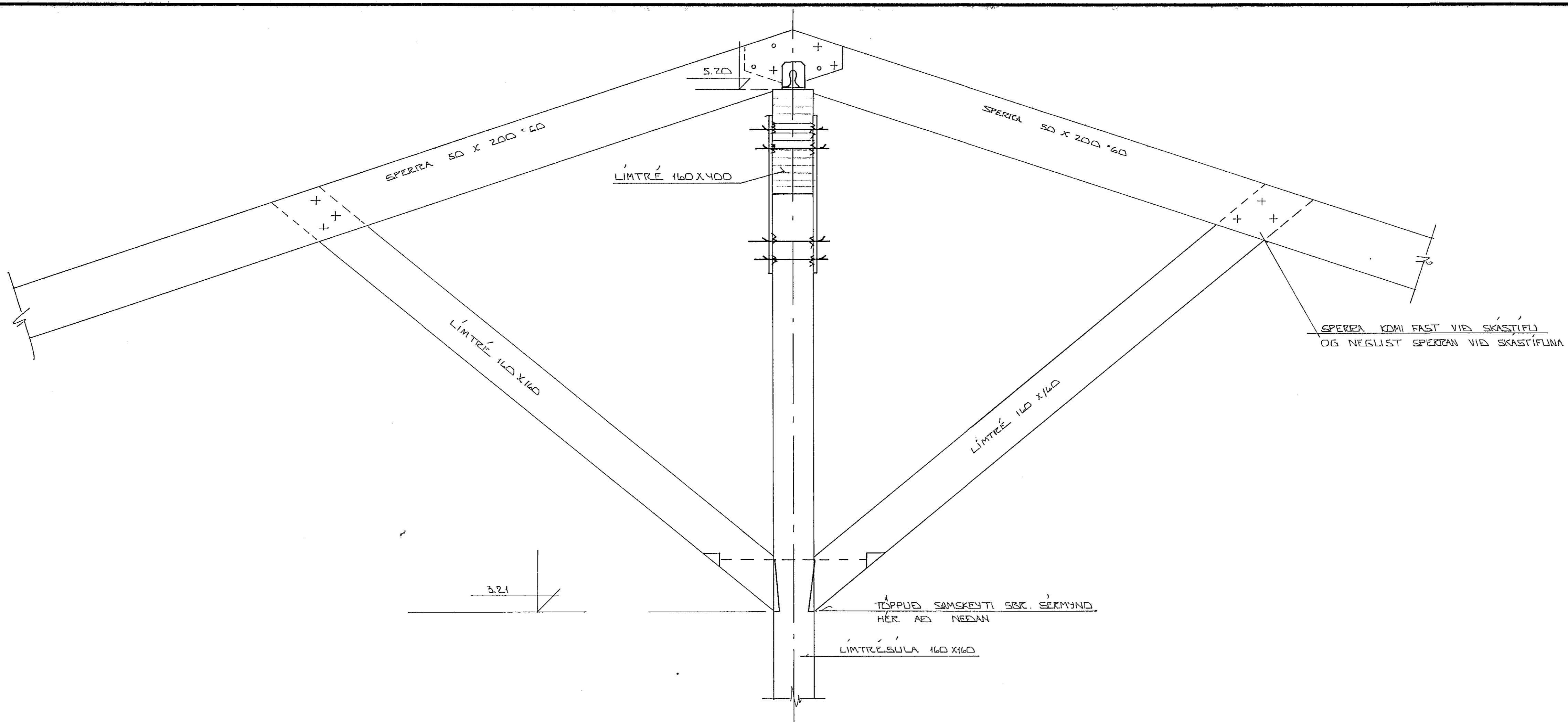
SÉRMYND 15 - 1:10
